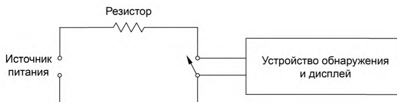
Рисунок 1 — Испытательная цепь отскока контактов
