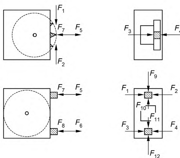
Рисунок 3e — Диск
