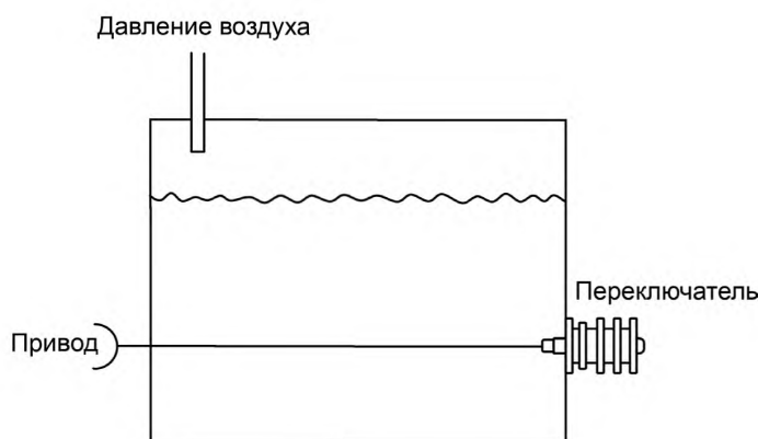
Рисунок 4 — Изолированная оболочка для погружения под давлением
