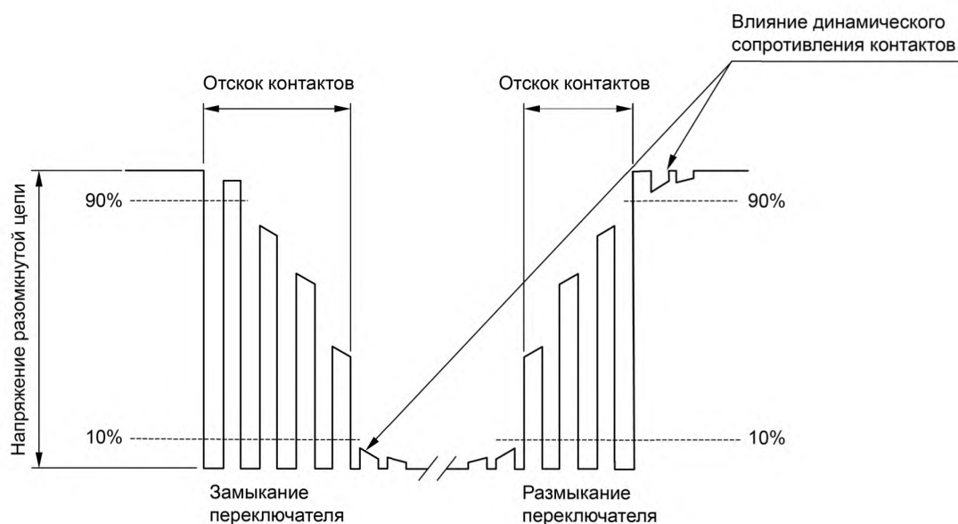
Рисунок 2 — Типичная схема отскока контактов
