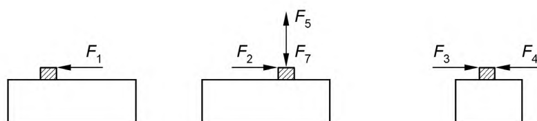
Рисунок 3c — Ползунок
