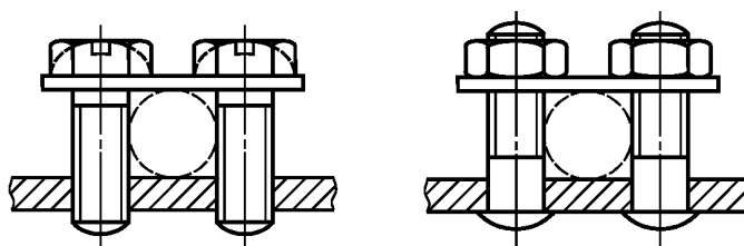
Рисунок 14е — Пластинчатые выводы
