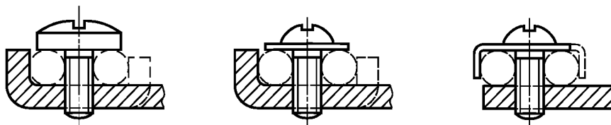
Рисунки 14b и 14c — Винтовые выводы
