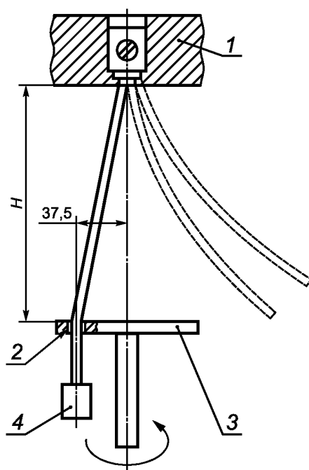
1 — фиксирующий узел; 2 — гильза; 3 — панель; 4 — груз
