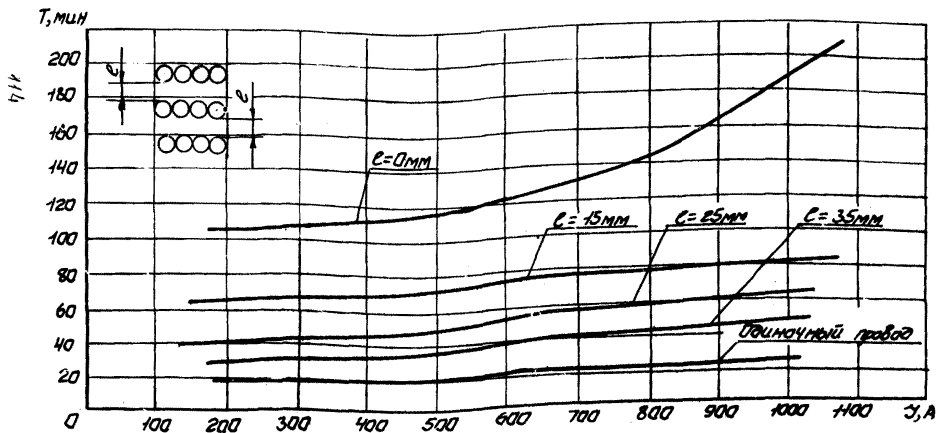
Рисунок Б.4- Зависимость постоянной времени наиболее нагретого провода в укладке 4x3 с горизонтальными зазорами e = 0 \text{ мм} , e = 15 \text{ мм} , e = 25 \text{ мм} , e = 35 \text{ мм} от тока нагрузки, t_0 = 40^\circ \text{C} , \gamma = 0,18 \text{ } \mu\text{C} , S = 240 \text{ мм}^2 .
