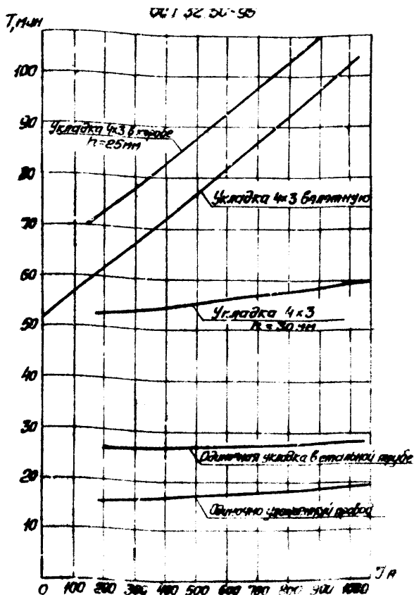
Рисунок Б.12 - Зависимость постоянной тока вольметра пробы от тока насыщения в случае укладки при t_0 = 40^\circ\text{C} , v = 0,43 \text{ м/с} , S = 135 \text{ мм}^2
