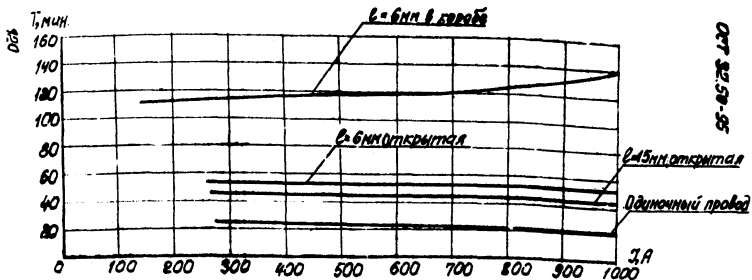
Рисунок В.10 - Зависимость постоянной времени наиболее нагретого провода в укладке 2x6, открытой с зазором l = 6 \text{ мм} , l = 15 \text{ мм} и в коробе ( l = 6 \text{ мм} ) от тока нагрузки, t_0 = 40^\circ \text{C} , V = 0.48 \text{ м/с} , S = 240 \text{ мм}^2
