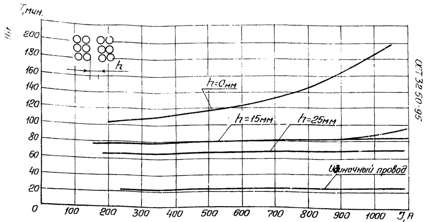
Рисунок Б.6 - Зависимость постоянной времени наиболее нагретого провода в укладке 4x3 с вертикальными зазорами h=0 мм, h=15 мм, h=25 мм от тока нагрузки, t_0=40^\circ\text{C} , v=0,48\text{ м/с} , S=240\text{ мм}^2
