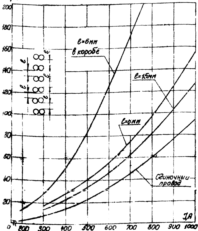
Рисунок 5.8 - зависимость установившихся температур наиболее нагретого провода в кладке 2.6 открытой с зазорами l=6\text{mm} , l=15\text{mm} и в коробе ( l=6\text{mm} ) от тока нагрузки, t_0=40^\circ\text{C} , V=0.48\text{ м/с} , S=240\text{ мм}^2
