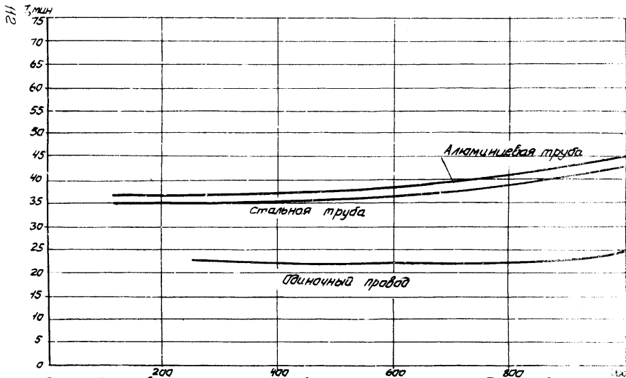
Рисунок Б.2 - зависимость постоянной времени от тока нагрузки для проводов, проложенного одиночно и в трубе (стальной или алюминиевой), t_0 = 40^{\circ}\text{C} , \nu = 0,48 \text{ м/с} , S = 240 \text{ мм}^2
