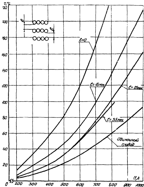
Рисунок Б.3— Зависимость установившихся перегревов наиболее нагретого провода в укладке 4 \times 3 с горизонтальными зазорами l=0 \text{ мм} , l=15 \text{ мм} , l=25 \text{ мм} , l=35 \text{ мм} от тока нагрузки, t_0=40^\circ\text{C} , \gamma=0,48 \text{ }^\circ\text{C}/\text{K} , S=240 \text{ мм}^2
