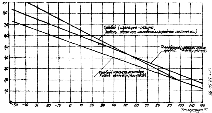
Рисунок Б13 - График зависимости между ресурсом и температурой теплобозных проводов (ТУ16-705.348-84)
