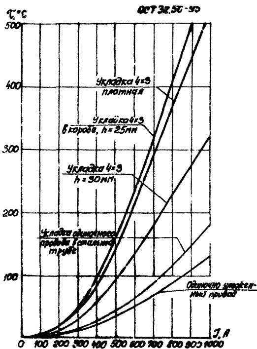
Рисунок Б11 - Зависимость установленной температуры проводов от тока нагрузки и способа укладки при t_{\text{в}} = 40^\circ\text{C} и \nu = 0,48\%/^\circ\text{C} , S = 185\text{ мм}^2
