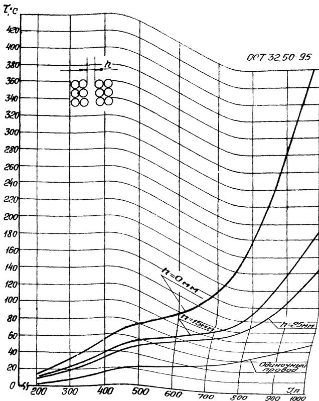
Рисунок Б.5.-Зависимость установившихся перепадов наиболее нагретого провода в укладке 4 \times 3 с вертикальными зазорами h=0\text{мм} , h=15\text{мм} , h=25\text{мм} , от тока нагрузки, t_v=40^\circ\text{C} , V=0,48\text{ м/с} , S=240\text{ мм}^2
