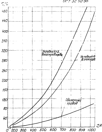
Рисунок Б.7- Зависимость установившихся перегревов наиболее нагретого провода в укладке 4x3 вплотную в коробе, t_0=40^\circ\text{C} , V=0,48\text{ м/с} , S=240\text{ мм}^2 117
