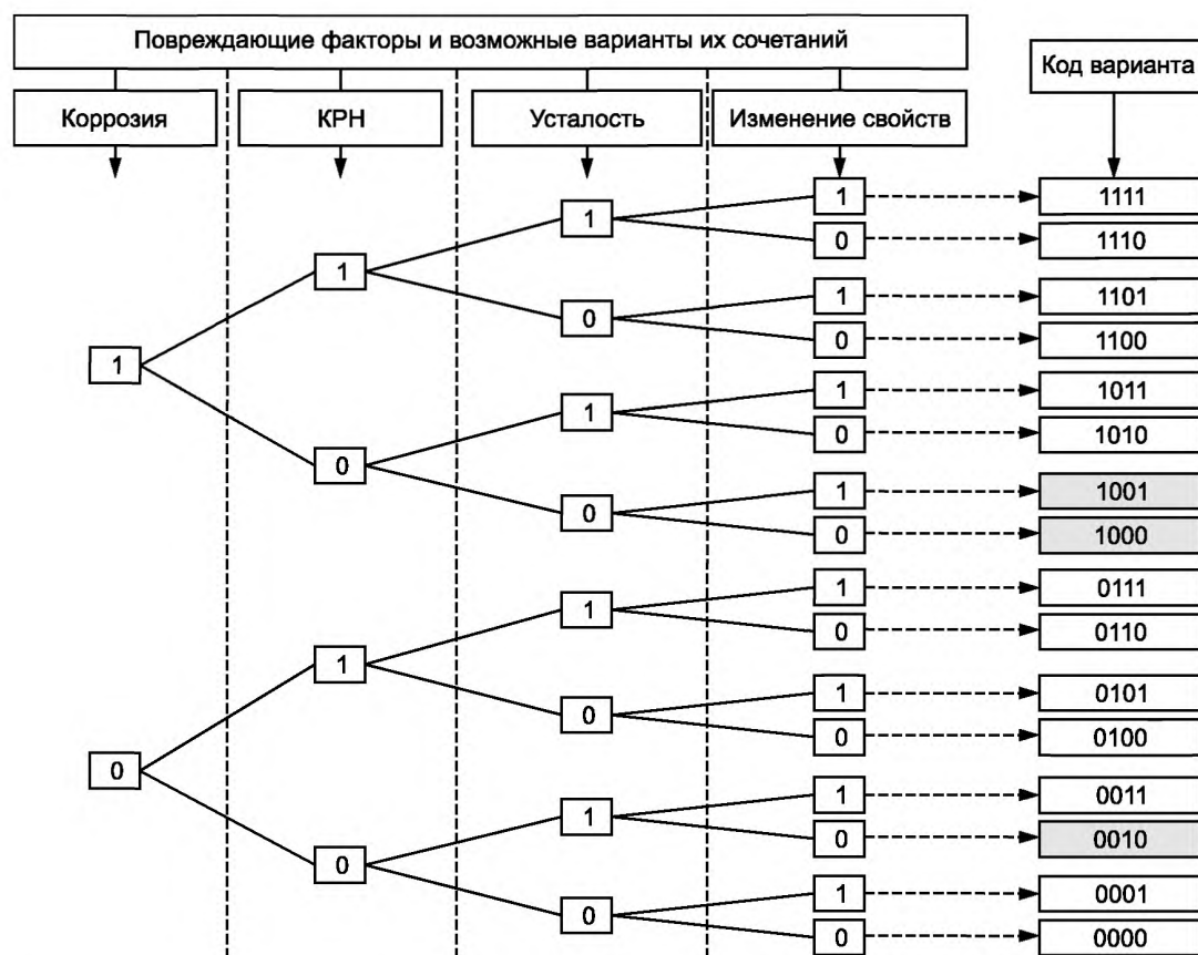
Рисунок Д.1 — Схема формирования вариантов учета механизмов накопления повреждений для оценки срока службы (ресурса) расчетного участка ЛЧМГ
