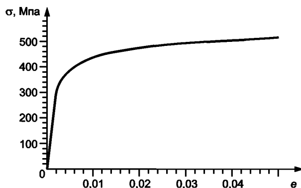
Рисунок Г.5 — Диаграмма статического деформирования для стали 09Г2С
