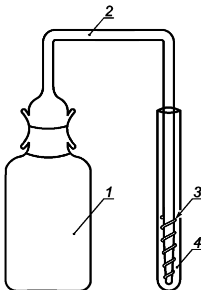
Рисунок 2 — Аппарат для отгонки мышьяка
