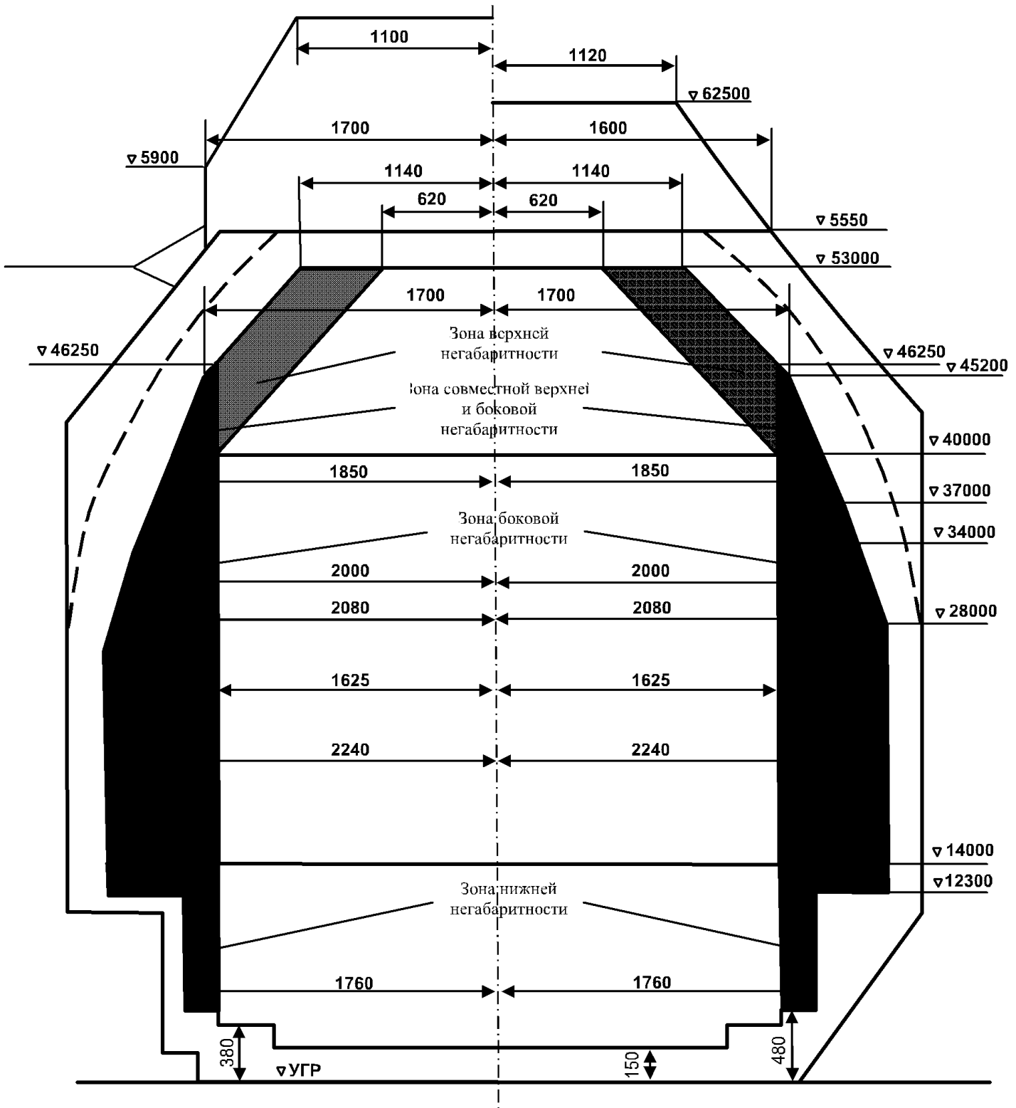
Рис.1. Зоны негабаритности груза
