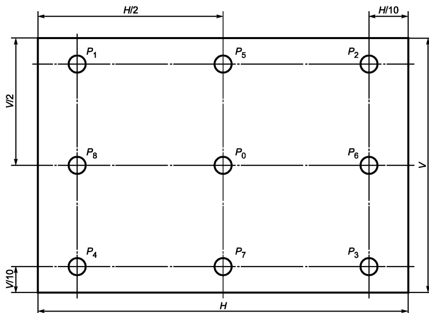
Рисунок 3 — Точки измерения
