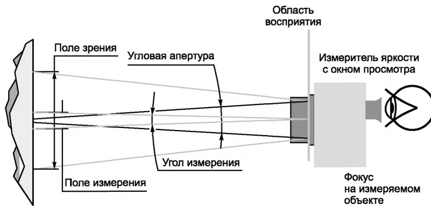
Рисунок 1 — Схема компоновки измерительной установки
