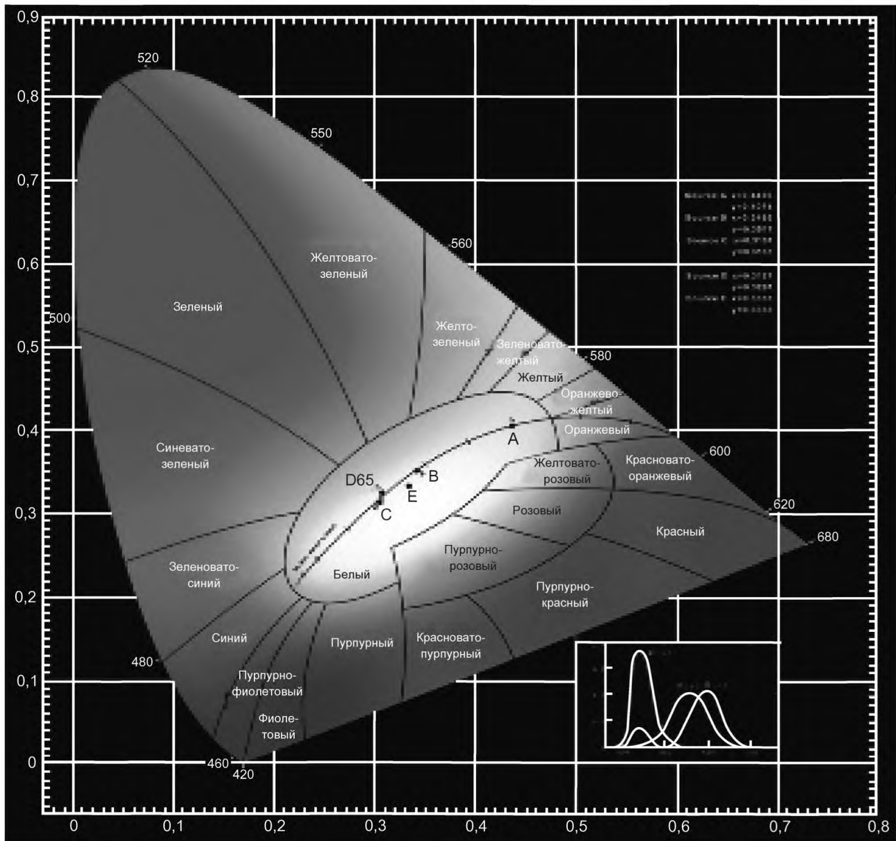
Рисунок D.1 — График цветности XYZ CIE 1931
