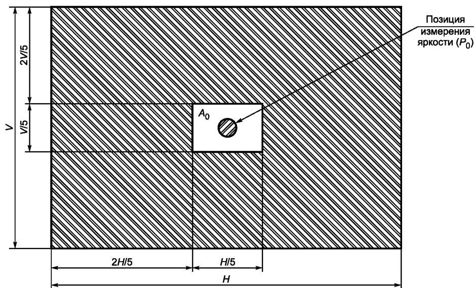
Шаблон для измерения яркости 4 % окна
