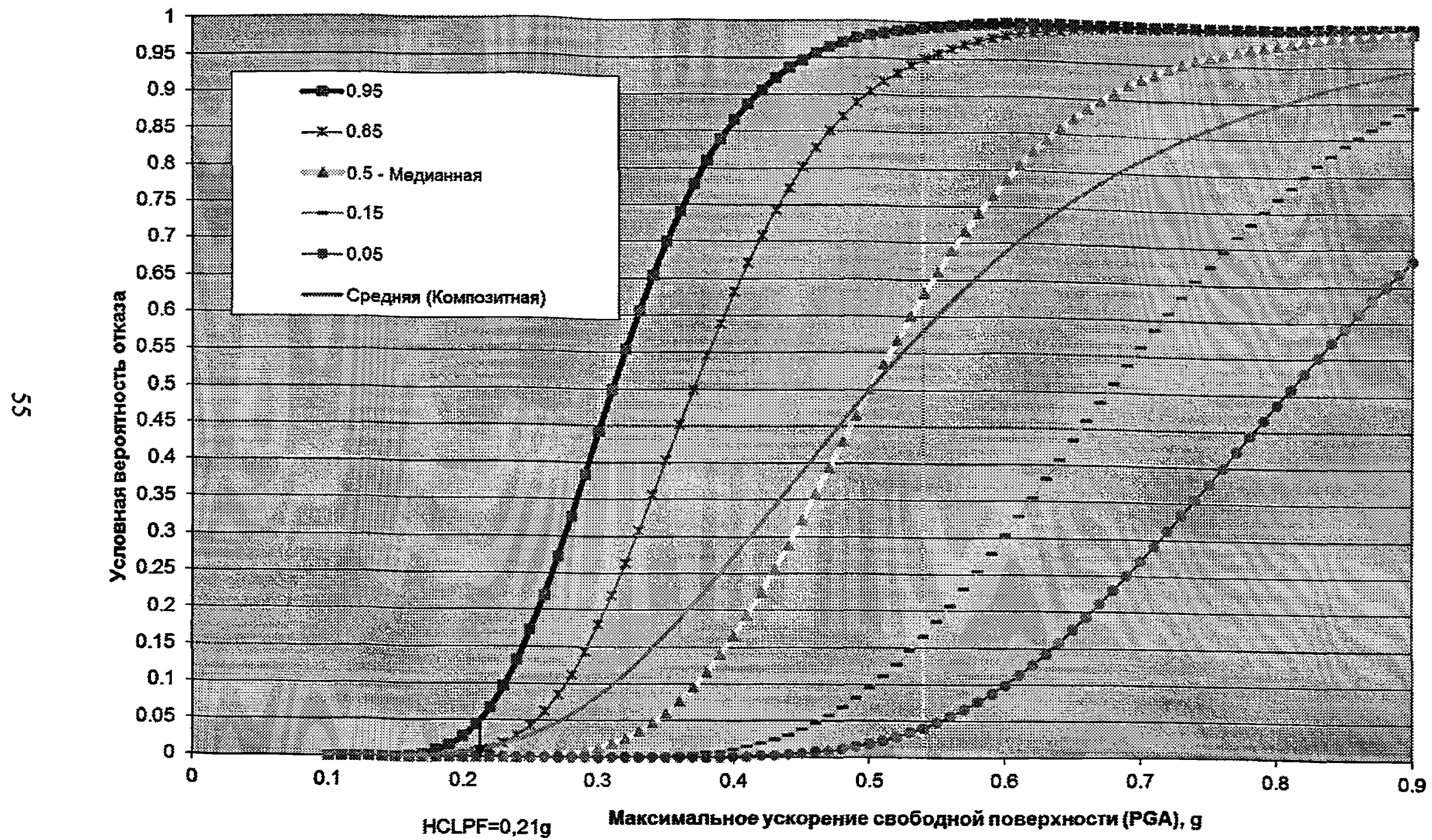
Рис. 7.2. Пример кривых сейсмической повреждаемости
