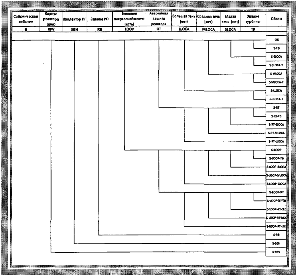
Рис. 8.1. Пример дерева сейсмических ИС
