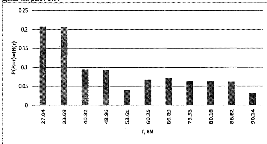
Рис. 6.9. Аппроксимация функции f_r(r) для источника № 1
