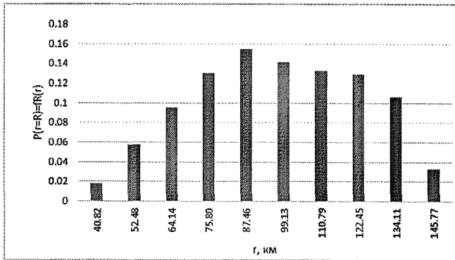
Рис. 6.10. Аппроксимация функции f_R(r) для источника № 2
