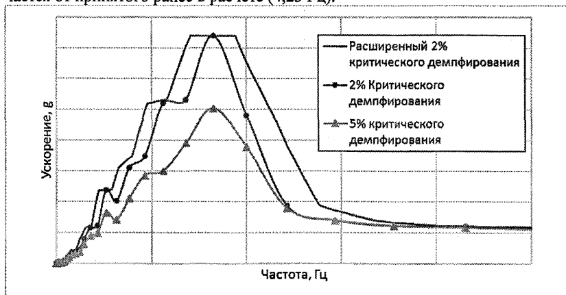
Рис. 7.5. Спектры ответа на отметке установки элемента
