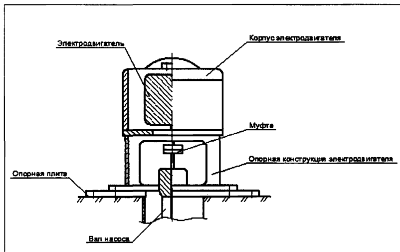
Рис. 7.3. Схема закрепления электродвигателя насоса
