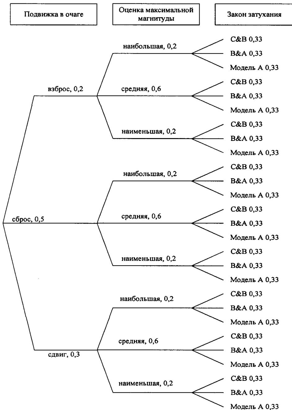
Рис. 6.2. Фрагмент логического дерева анализа неопределенности
