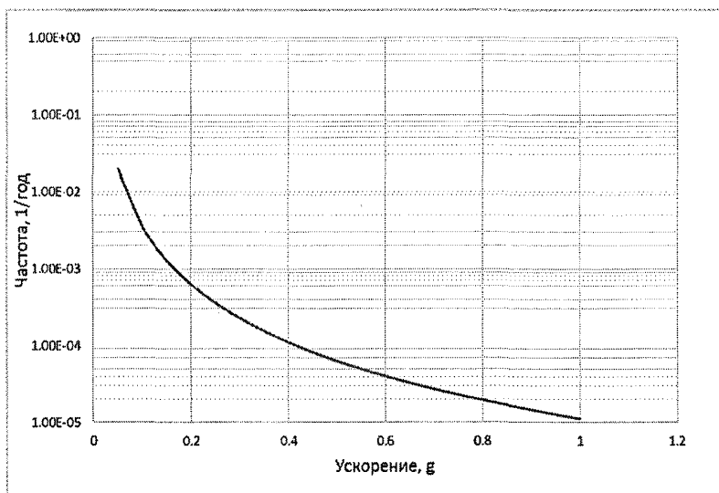
Рис. 6.8. Кривая опасности для примера с точечным источником
