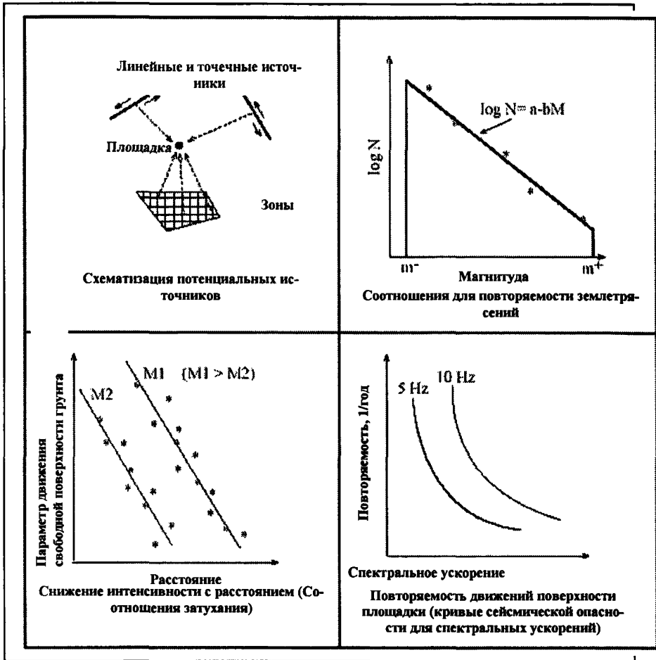
Рис. 6.1. Основные этапы вероятностного анализа сейсмической опасности площадки
