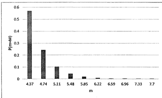
Рис. 6.11. Гистограмма P(m = M) для 10 интервалов магнитуд
