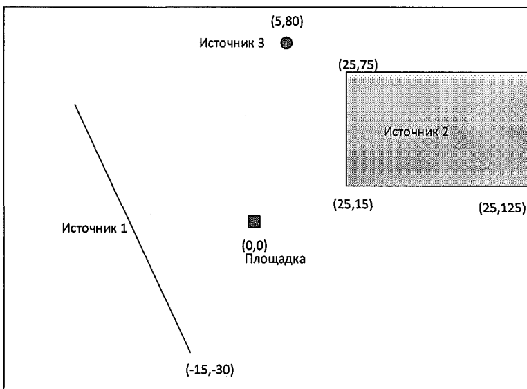
Рис. 6.9. Модель с тремя источниками
