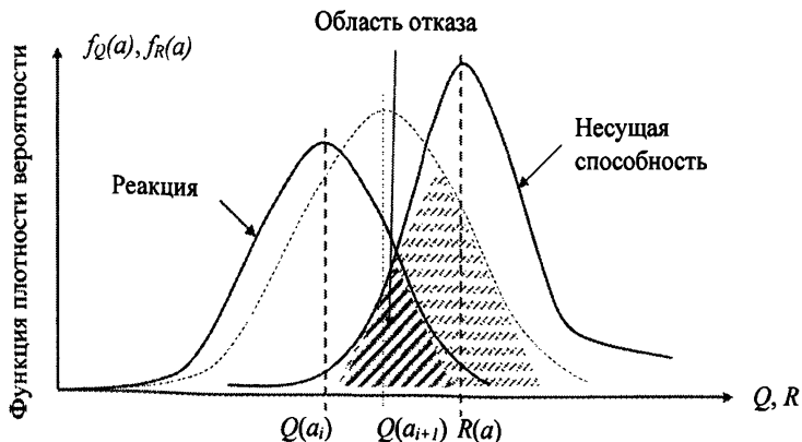
Рис. 7.1. Комбинация значений реакции и сейсмической повреждаемости, приводящая к отказу элемента
