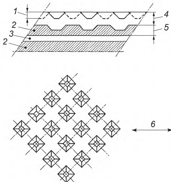
Рисунок 1 — Полости для смазки в опорах типа D
