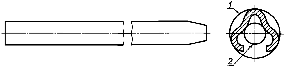
1 — наружный диаметр; 2 — минимальный внутренний диаметр
