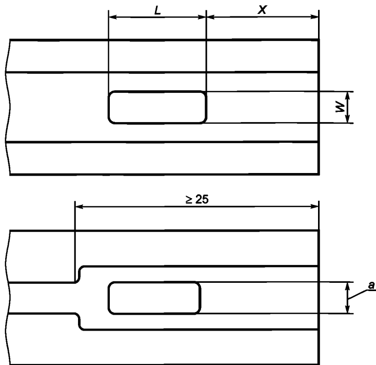
a — Дополнительный линейный слот под крюк-экстрактор
