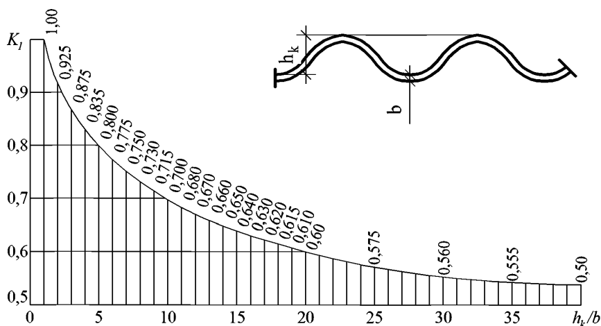
Рисунок 6.6 — График для определения коэффициента K_1
