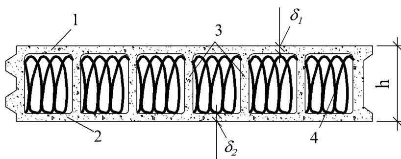
1, 2 — полки панели; 3 — ребра панели; 4 — утеплитель
