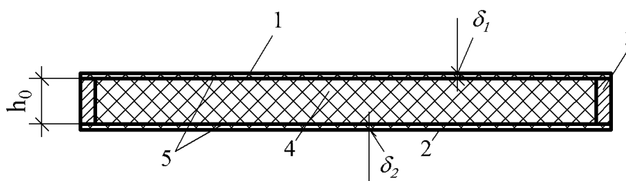
1, 2 — асбестоцементные обшивки; 3 — элементы обрамления панели; 4 — заполнитель (пенопласт); 5 — клеевой шов
