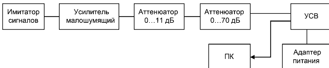
Рисунок В.3 — Схема определения чувствительности модуля ГНСС
