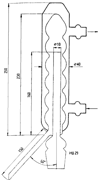
Рис. 7. Насадка для перегонки с водяным паром (НШ 29 – нормальный шлиф) (размеры в мм).
