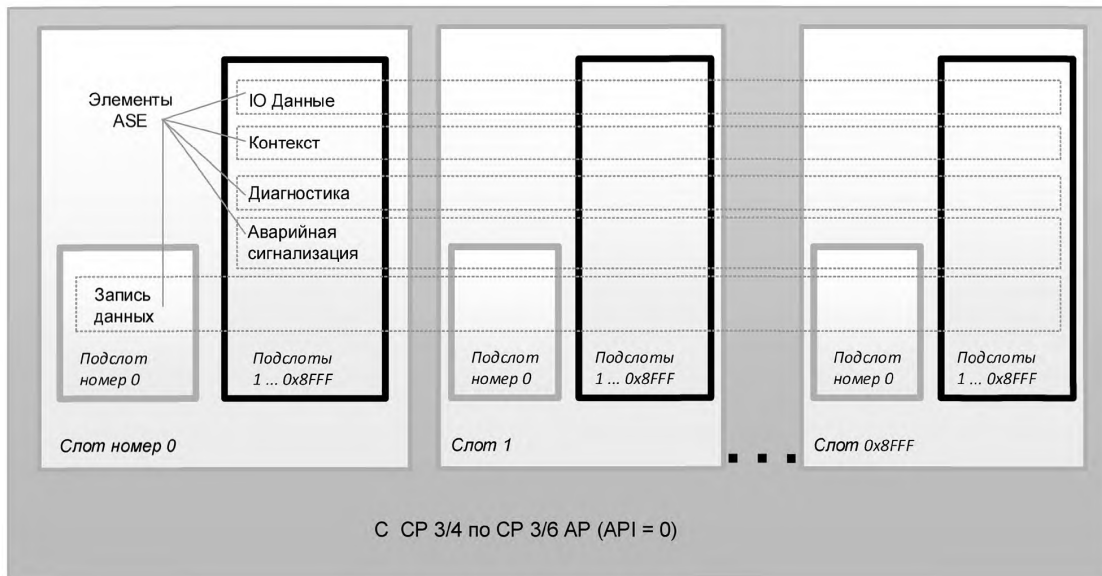
Рисунок 13 — Модель устройства
