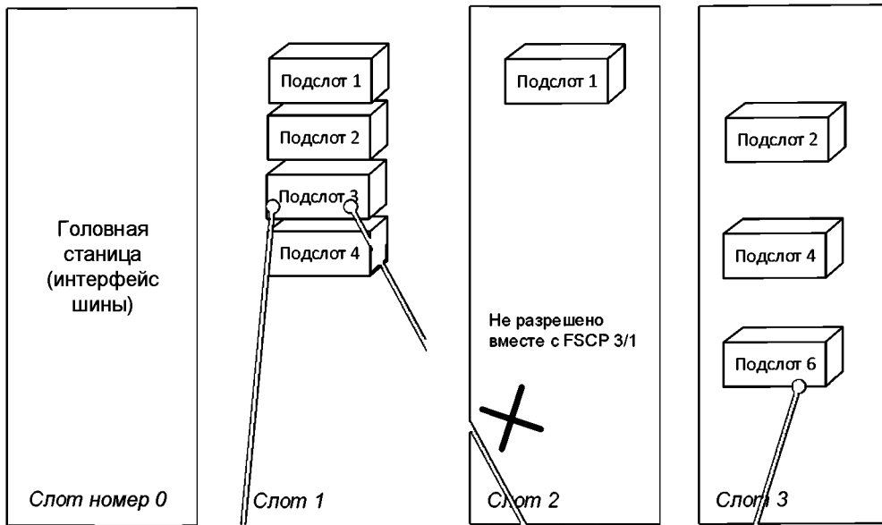
Модульное ИО устройство
