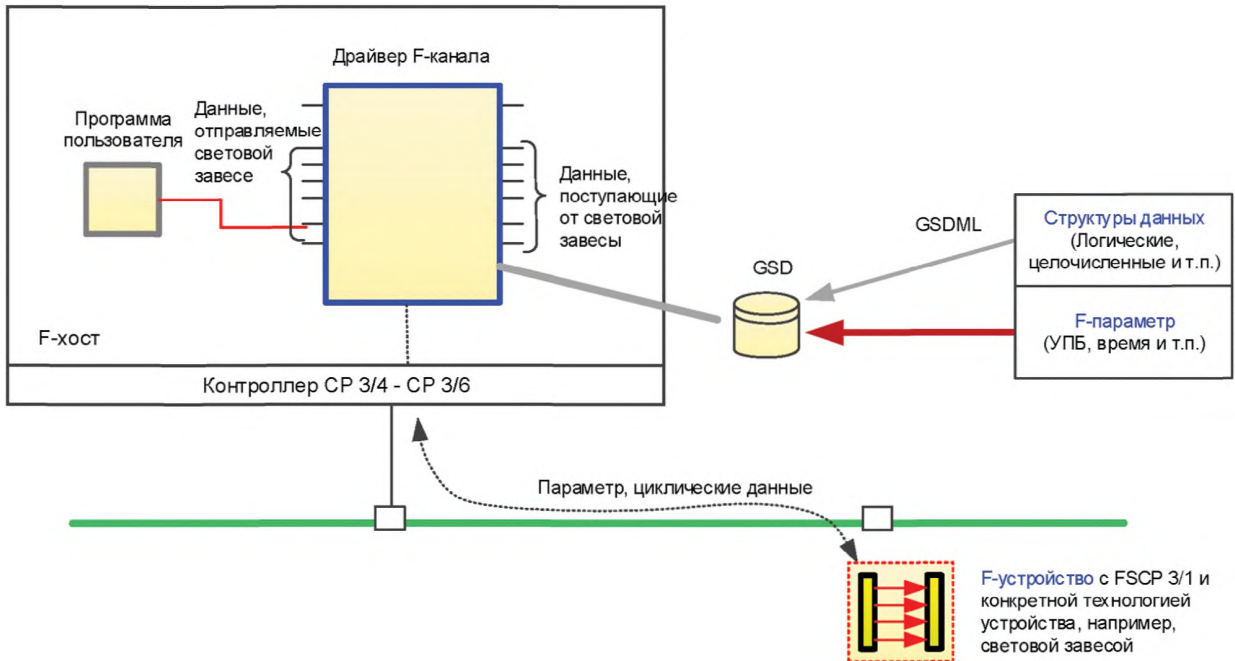
Рисунок б1 — Драйвер F-канала в качестве «клея» между F-устройством и пользовательской программой
