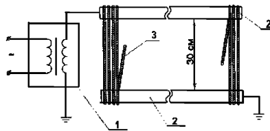
Рис. 3. Схема электрических испытаний изолирующего каната: 1 - источник испытательного напряжения; 2 - металлическая труба; 3 - испытываемый изолирующий канат
