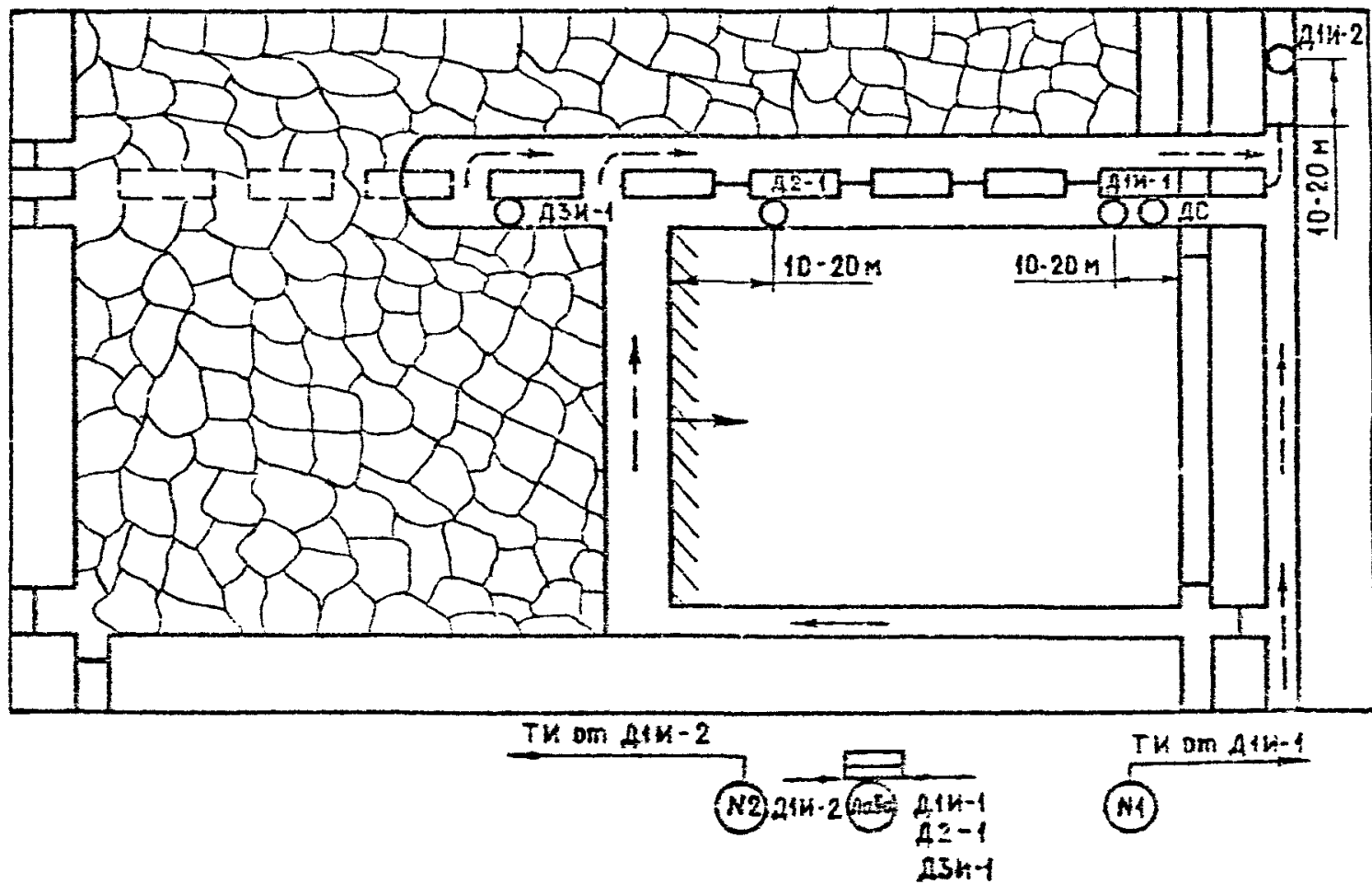
Рис.24. Схема размещения аппаратуры АГП при системе разработки длинными столбами по простиранию с применением дренажного штрэка и смесительной камеры
