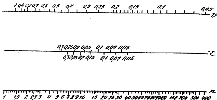
Рис. 2. Номограмма для определения точности среднего (нормальное распределение, \beta = 0,90 и \beta = 0,95 )
