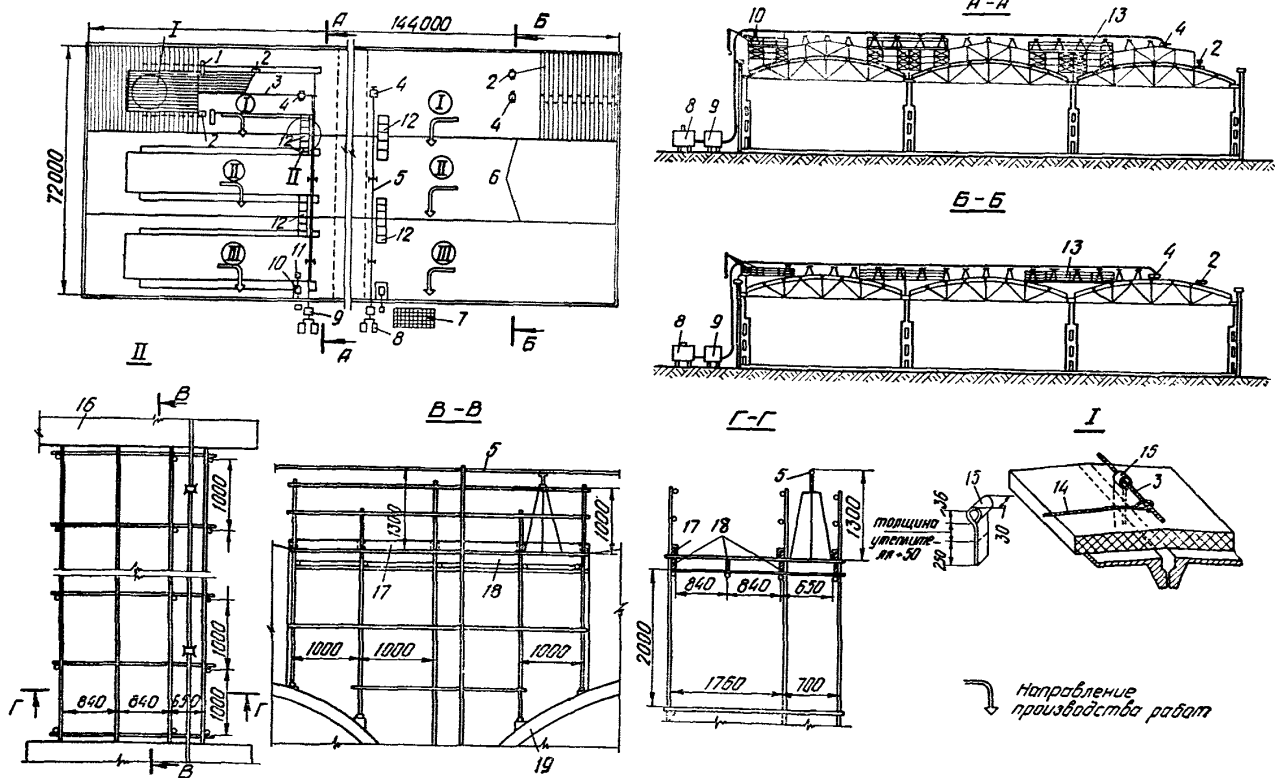
Рис. Организация работ на корпусе
