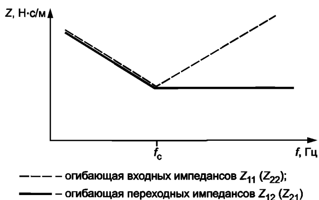
Рисунок А.1 — Виброизолятор, нагруженный массой машины
