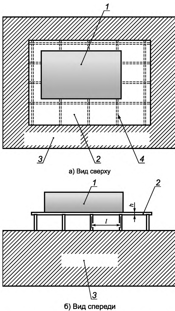
Рисунок А.8 — Схематическое изображение нагруженной фундаментной плиты
