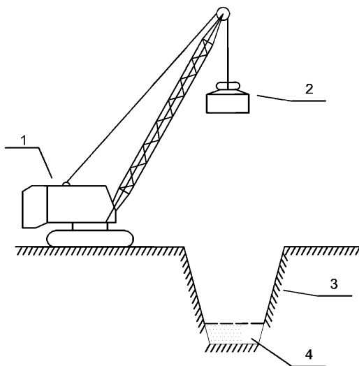
1- грузоподъемный механизм; 2-трамбовка; 3- шурф; 4- уплотняемый грунт.
