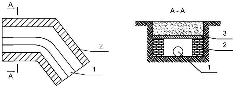
Рисунок 3 - Устройство непроходного канала
