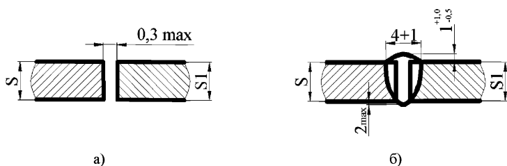
а) подготовка кромок; б) сварной шов
