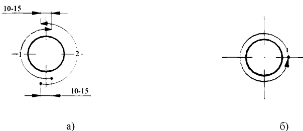
Рисунок 7- Схема выполнения сварного неповоротного шва
