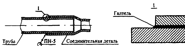
Рисунок 3 – Конструкция паяного соединения ПН-5
