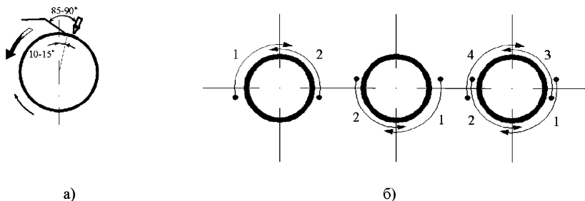
а) с поворотом на 360°; б) в два поворота на 180°
