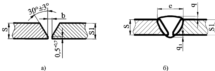
а) подготовка кромок под сварку; б) сварное соединение
