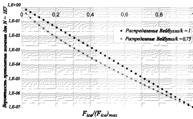
Рис.10.7.5.1.8 Распределение Вейбулла
