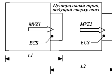
Рис. 2.2.1.2-1 Эвакуационный трап обслуживает одну главную вертикальную зону
