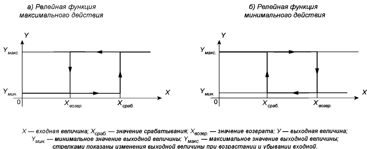
Рисунок 1 — Графики релейных функций одной входной величины
