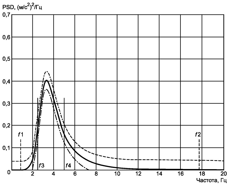
Рисунок 9 — PSD для входного спектрального класса EM 8 (мини-погрузчик \leq 4\,500 кг)
