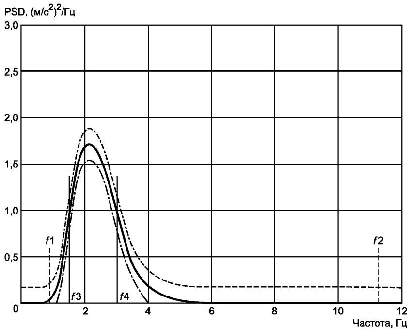
Рисунок 4 — PSD для входного спектрального класса EM 3 (колесный погрузчик > 4 500 кг)
