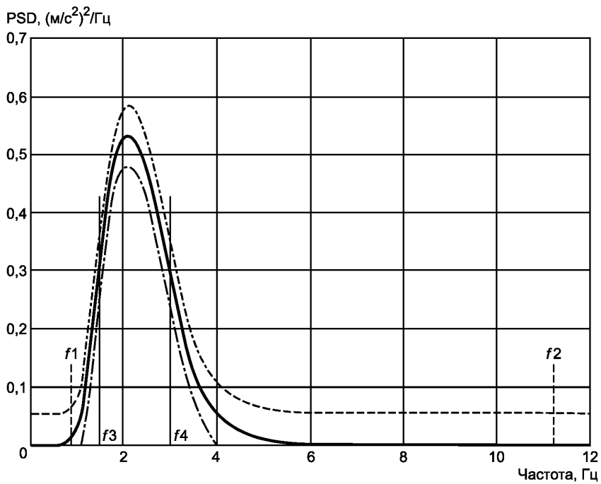
Рисунок 5 — PSD для входного спектрального класса EM 4 (грейдер)
