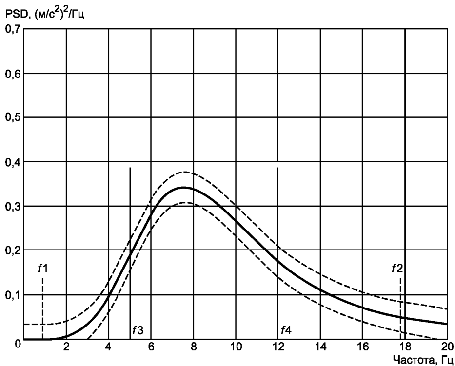
Рисунок 7 — PSD для входного спектрального класса EM6 (гусеничный землевоз, гусеничный погрузчик, гусеничный бульдозер ≤ 50 000 кг)
