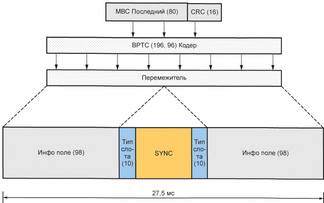
Рисунок А.28 — Формат последнего блока MBC сообщения
