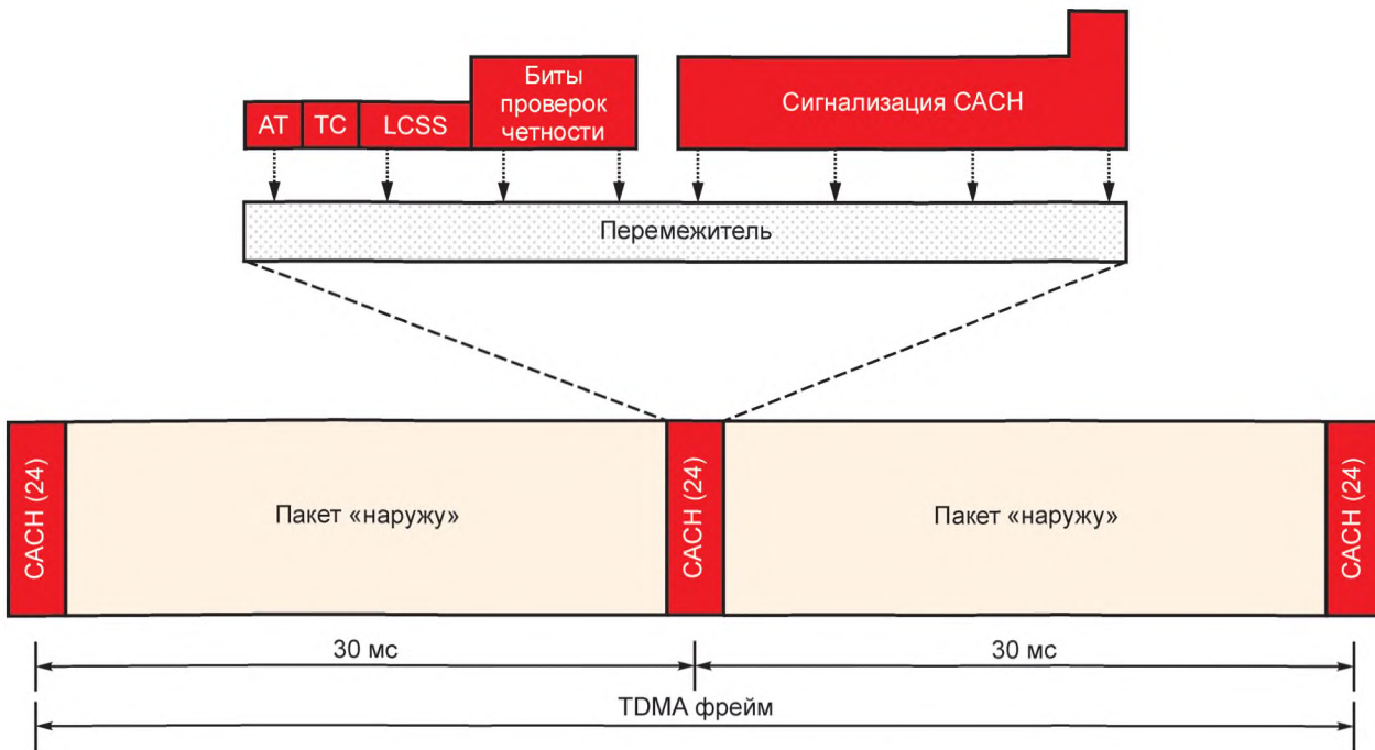
Рисунок А.17 — Формат пакета CACH
