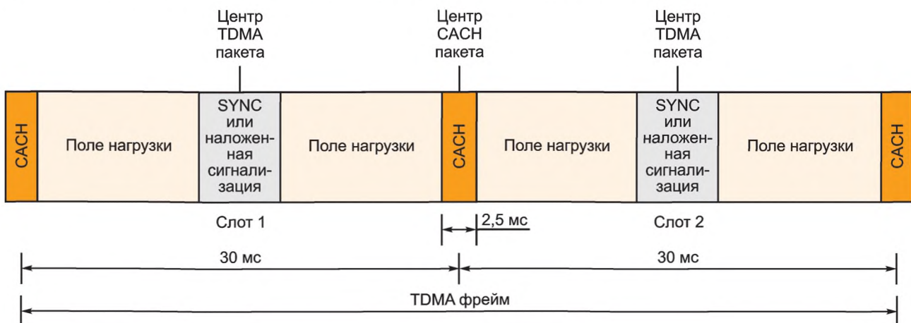
Рисунок А.5 — Структура TDMA фрейма от источника БС
