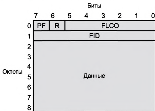
Рисунок А.20 — Общая структура полного LC сообщения
