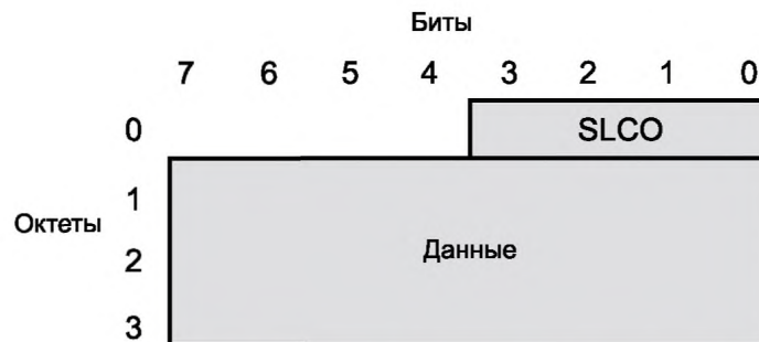
Рисунок А.21 — Структура короткого LC сообщения
