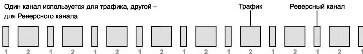
Рисунок А.9 — Канал трафика с защитным интервалом
