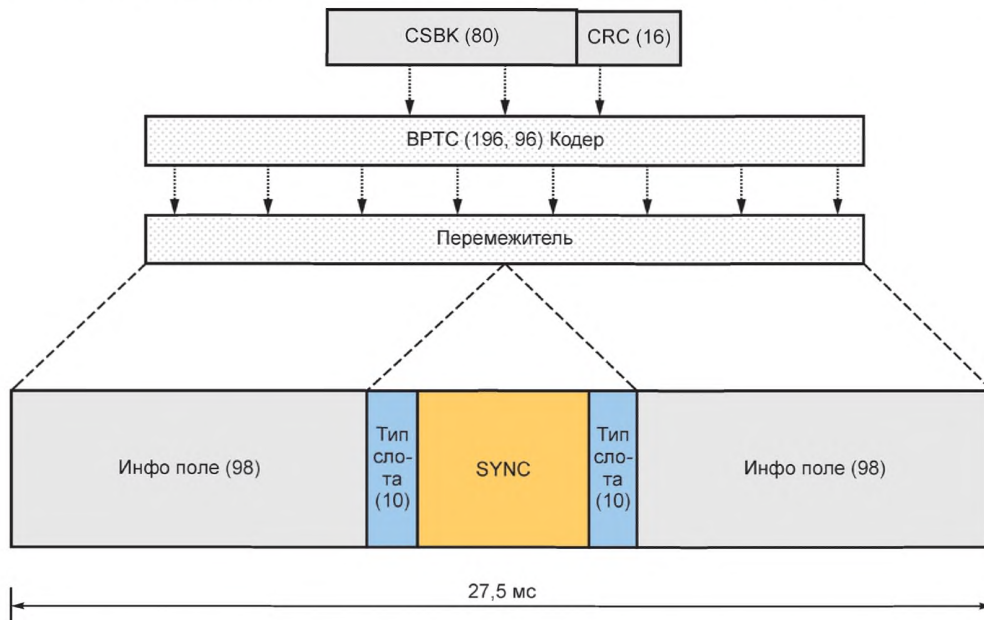
Рисунок А.25 — Формат сообщения блока управления сигнализацией (CSBK)
