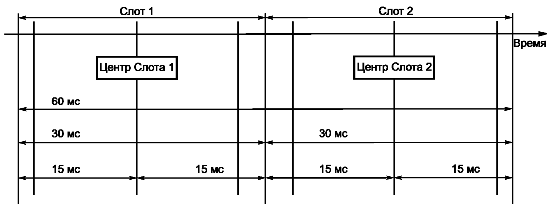
Рисунок А.12 — Синхронизация TDMA фрейма
