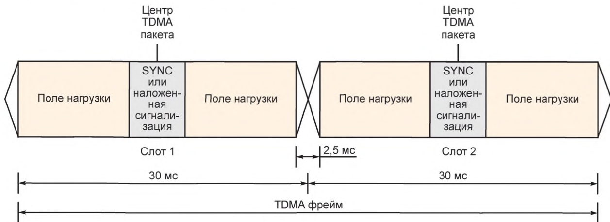
Рисунок А.4 — TDMA фрейм от источника МС
