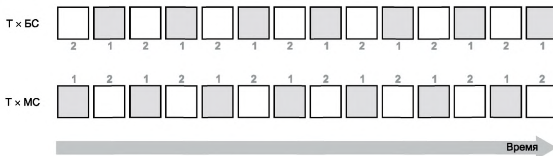
Рисунок А.14 — Синхронизация канала со сдвигом
