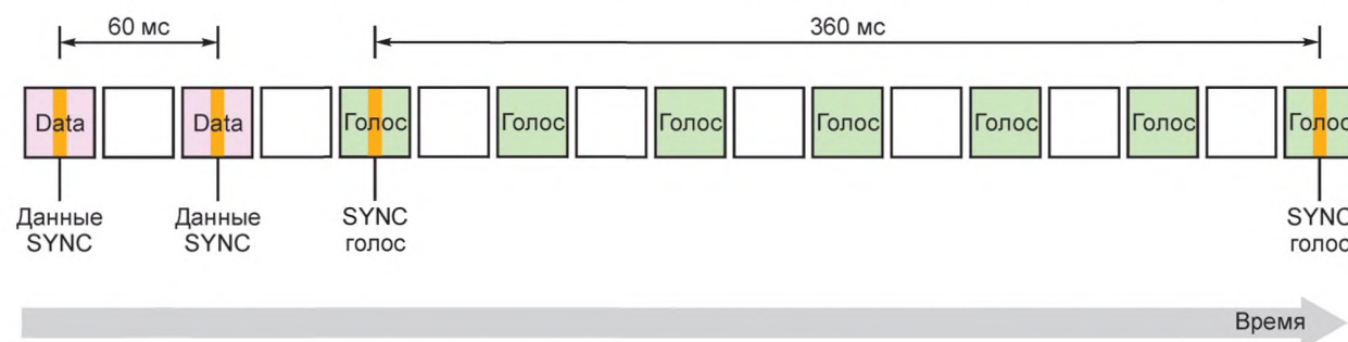
Рисунок А.6 — Синхронизация канала от МС к БС
