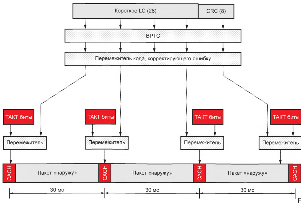
Рисунок А.24 — Короткое LC сообщение в составе CACH
