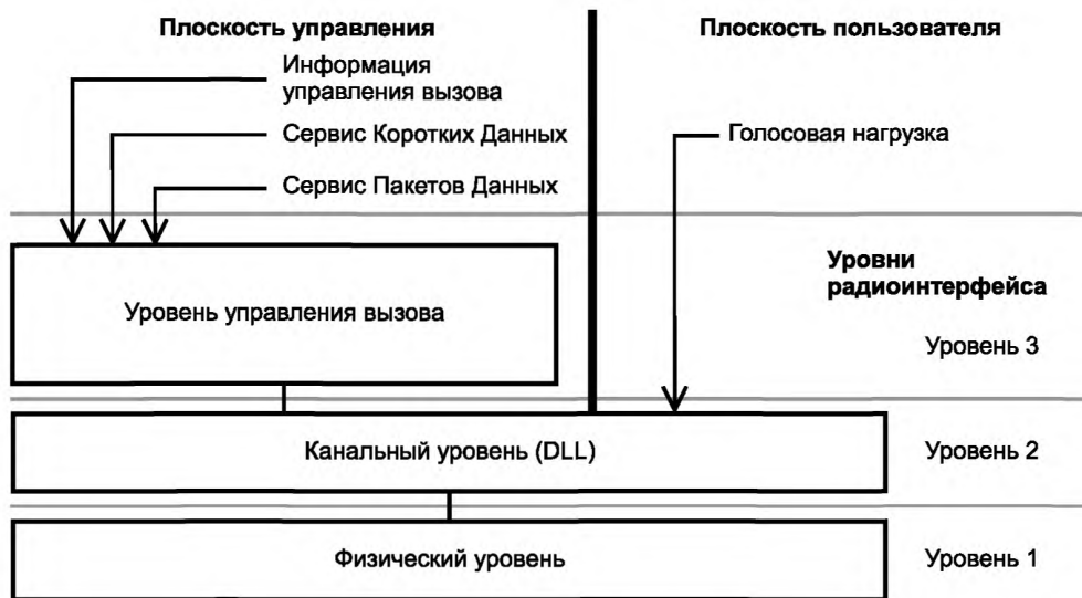
Рисунок А.1 — Стек протоколов DMR
