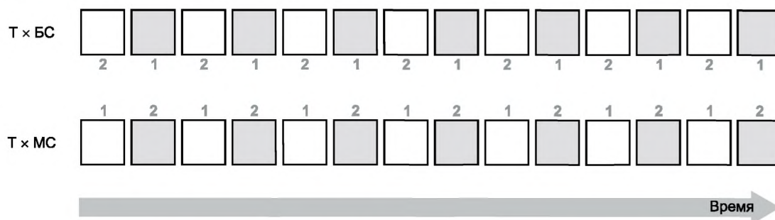
Рисунок А.13 — Диаграмма выровненной синхронизации канала
