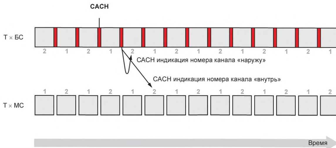
Рисунок А.8 — Синхронизация пакета CACH для индикации номера канала
