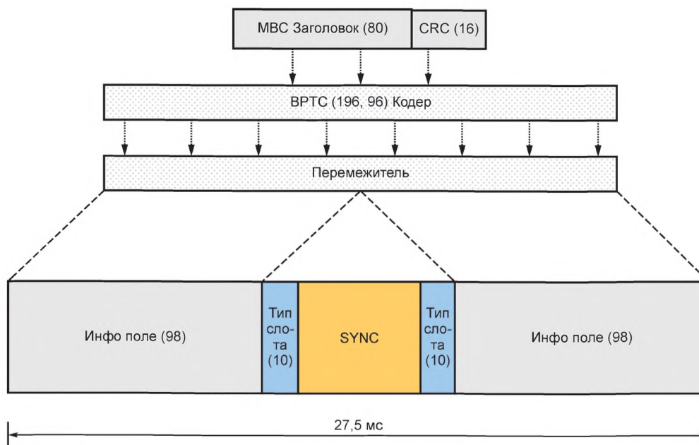
Рисунок А.26 — Формат пакета MBC заголовка сообщения
