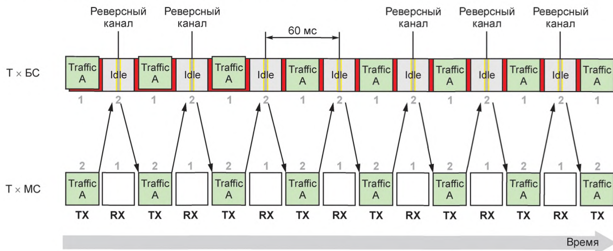
Рисунок А.15 — Синхронизация назначенного реверсивного канала
