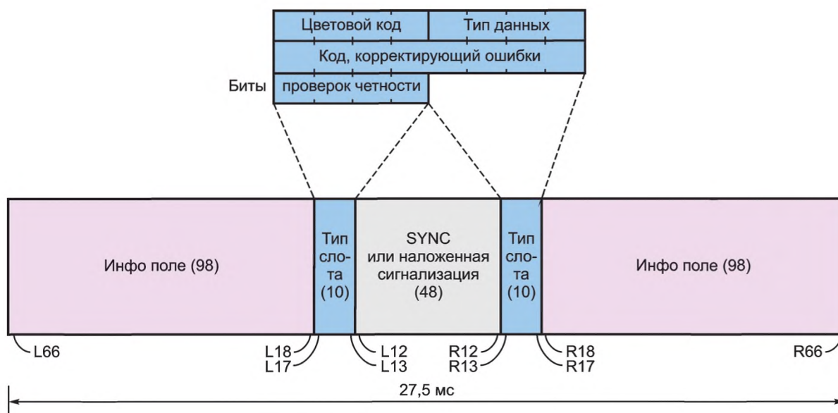
Рисунок А.16 — Формат пакета общих данных
