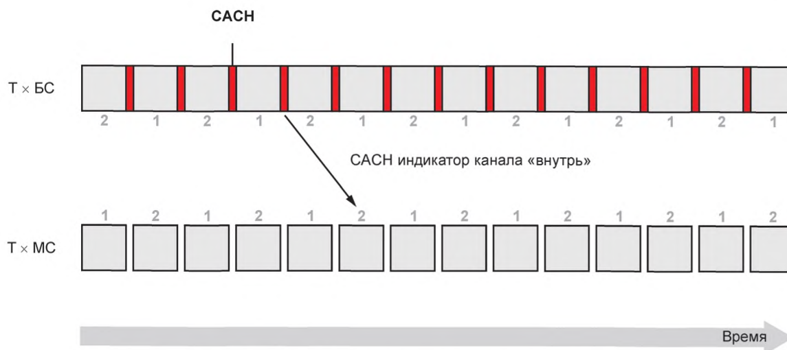
Рисунок А.7 — Синхронизация между пакетами CACH и «внутри»
