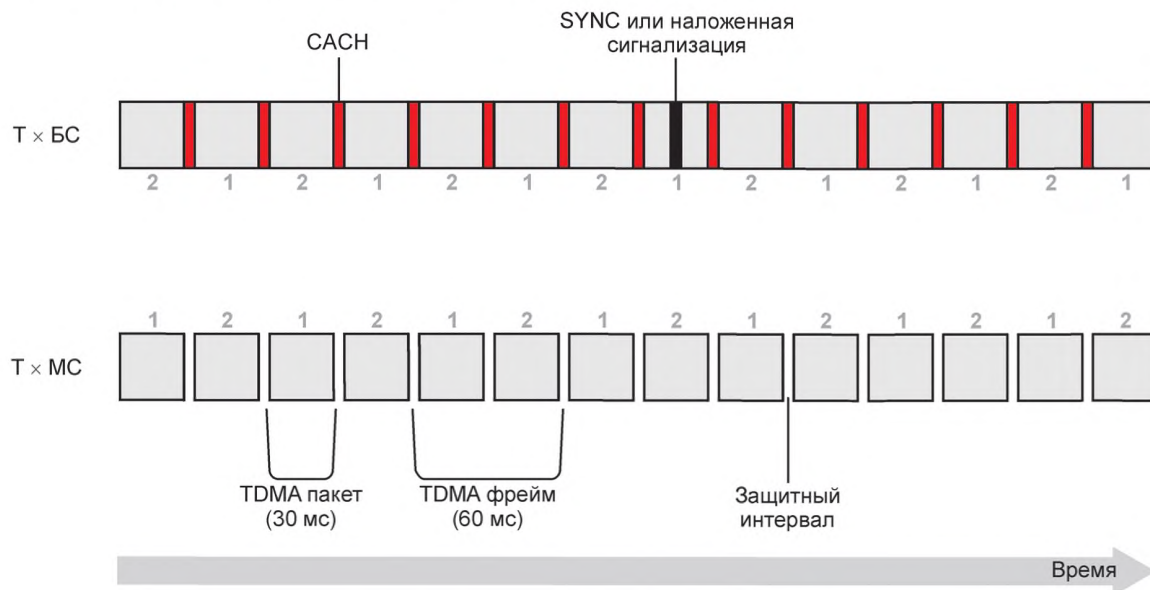
Рисунок А.2 — Диаграммы обмена между БС и МС
