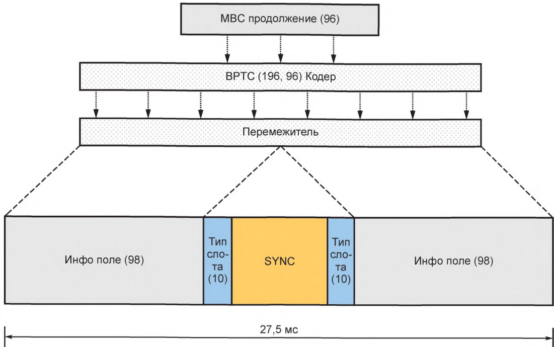
Рисунок А.27 — Формат пакета промежуточного MBC сообщения
