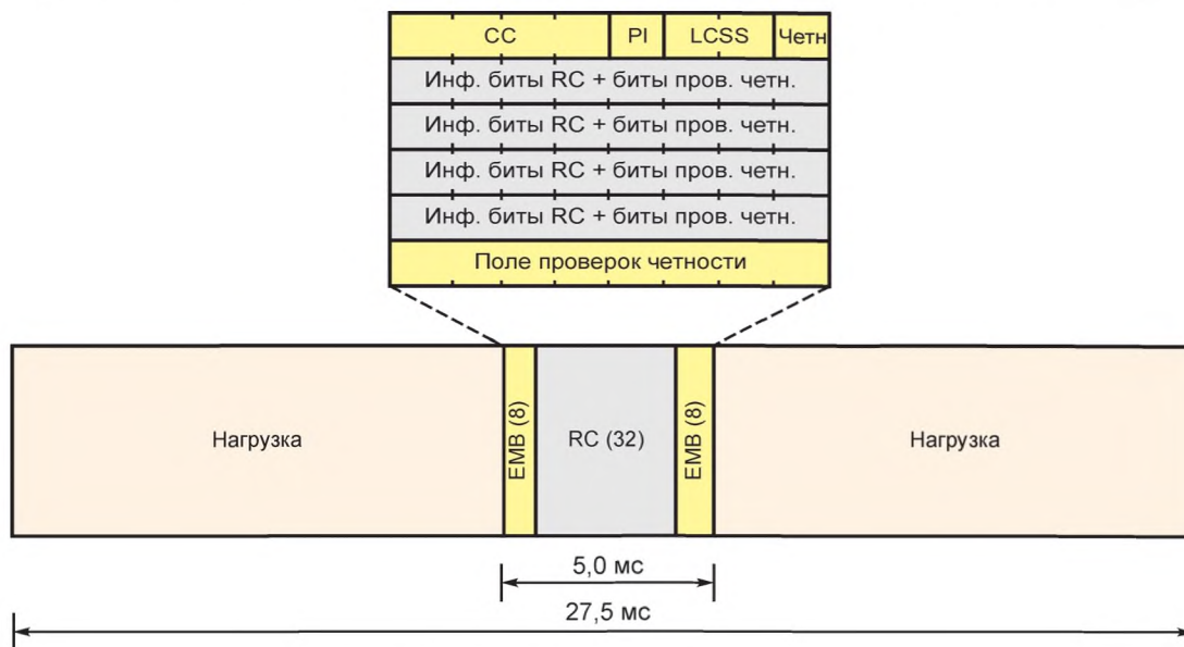
Рисунок А.19 — Формат пакета реверсного канала
