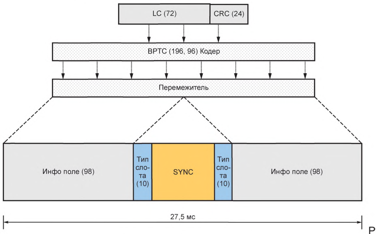
Рисунок А.22 — Формат LC пакета голосового заголовка
