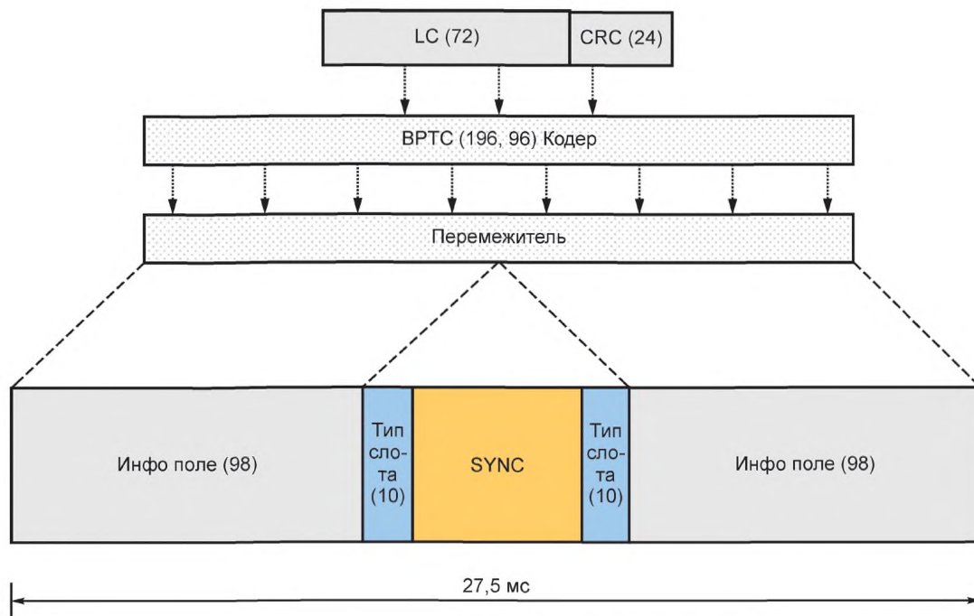
Рисунок А.23 — Формат пакета «Окончание LC»
