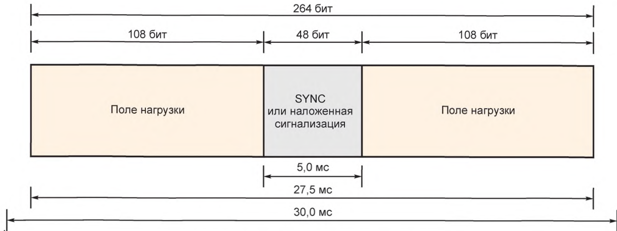
Рисунок А.3 — Общая структура пакета
