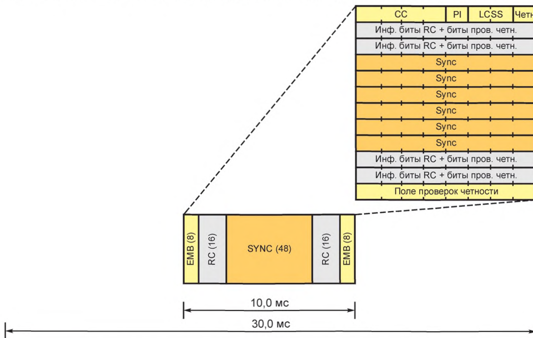
Рисунок А.18 — Формат автономного пакета направления «внутри» RC канала
