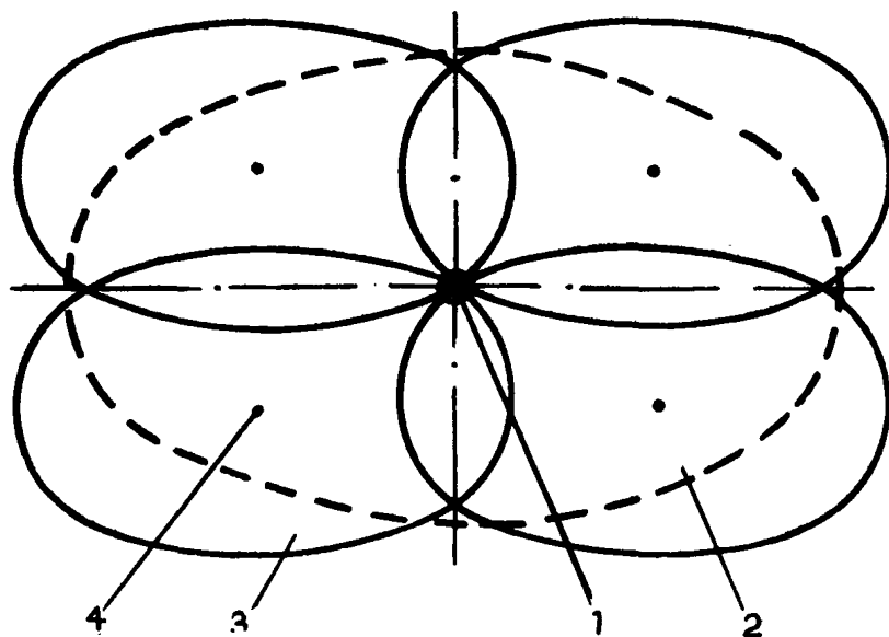
Рис. 8. Схема определения количества точек нагнетания (тампонажных скважин) на примере расчета параметров формирования изоляционной завесы в интервале водоносного горизонта 681—717 м: 1 — проектируемый шахтный ствол; 2 — контур расчетной изоляционной завесы ( R_2=42,0 м, R_1=26,3 м.); 3 — контур распространения тампонажного раствора из отдельной скважины ( r_2=28,2 м, r_1=17,5 м); 4 — точки нагнетания (тампонажные скважины).
