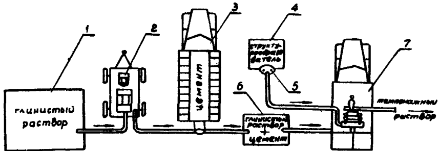
Рис. 4. Принципиальная технологическая схема приготовления глиноцементных тампонажных растворов: 1 — емкость-накопитель глинистого раствора; 2 — насос; 3 — смесительная машина; 4 — емкость со структурообразователем; 5 — насос для подачи структурообразователя; 6 — емкость; 7 — тампонажный насос.
