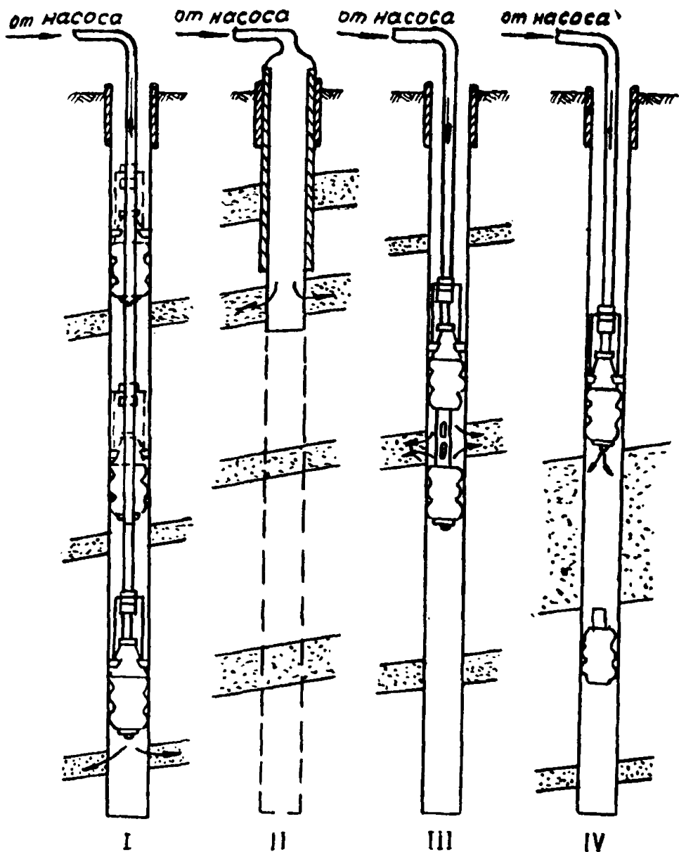
Рис. 6. Технологические схемы нагнетания:
