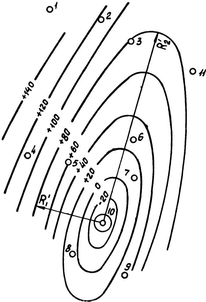
Рис. 3. План гидроизогипс в зоне возмущающей скважины.
