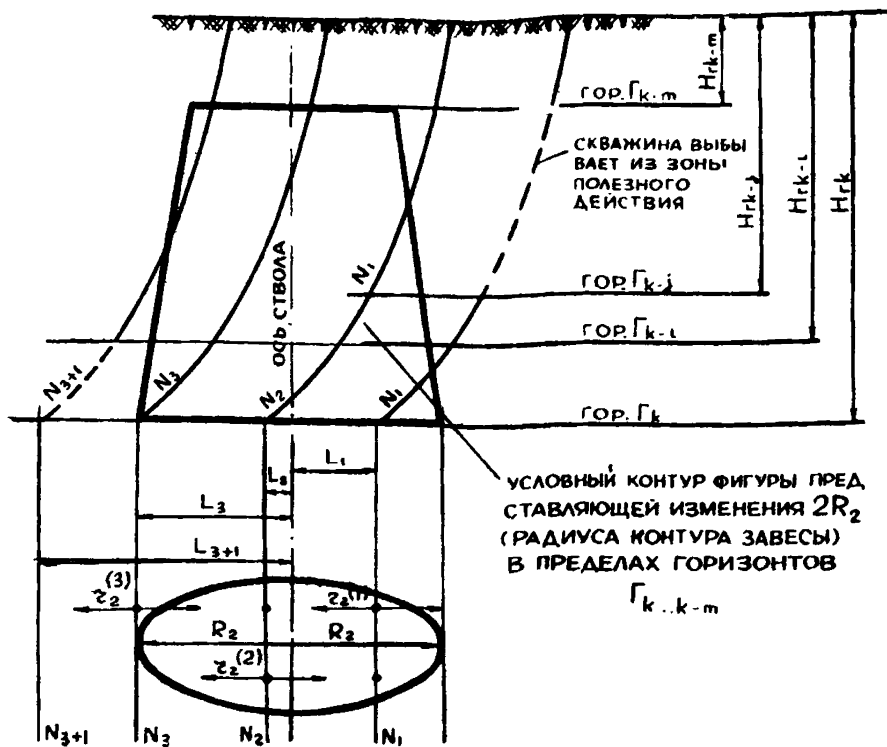
Рис. 11. Принципиальная схема привязки тампонажных скважин.
