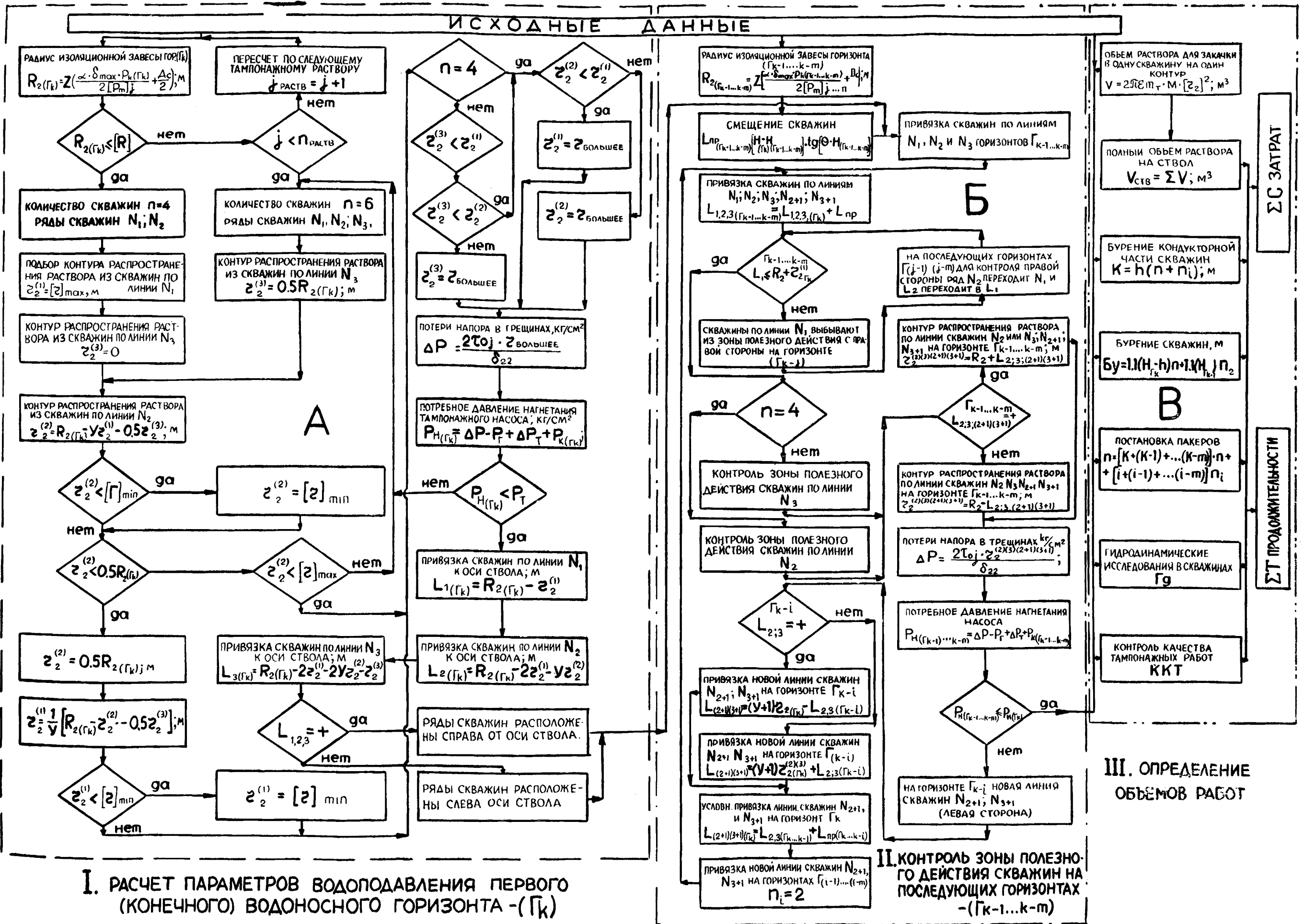
Рис. 10. Логико-информационная модель расчета параметров водоподавления комплексным методом.
