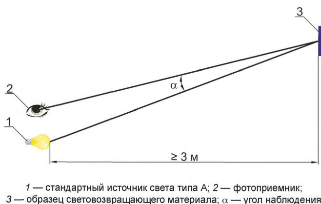
Рисунок Б.1 — Схема измерения удельного коэффициента световозвращения (вертикальный угол наблюдения)
