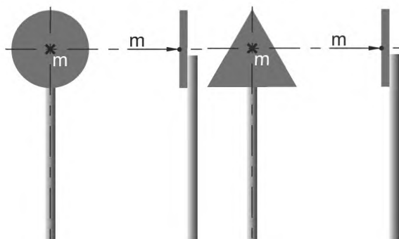
Рисунок А.1 — Схема приложения расчетной ветровой нагрузки
