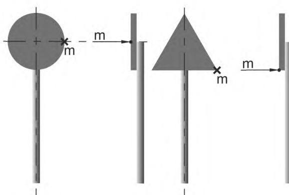
Рисунок А.4 — Схема приложения горизонтальной точечной нагрузки
