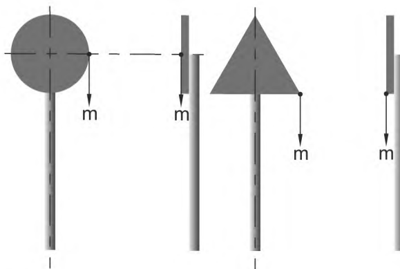
Рисунок А.3 — Схема приложения вертикальной точечной нагрузки
