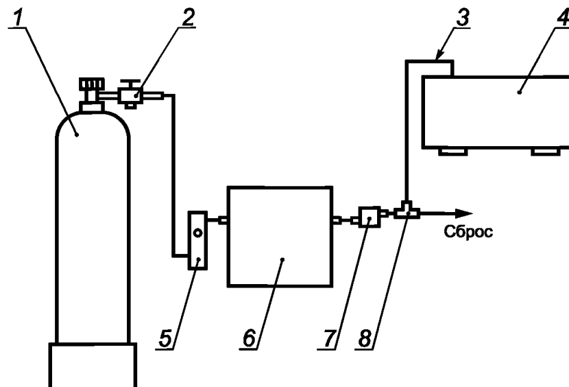
Рисунок Б.1 — Газовая схема для подачи ГС от генератора со встроенным побудителем расхода на газоанализатор-компаратор
