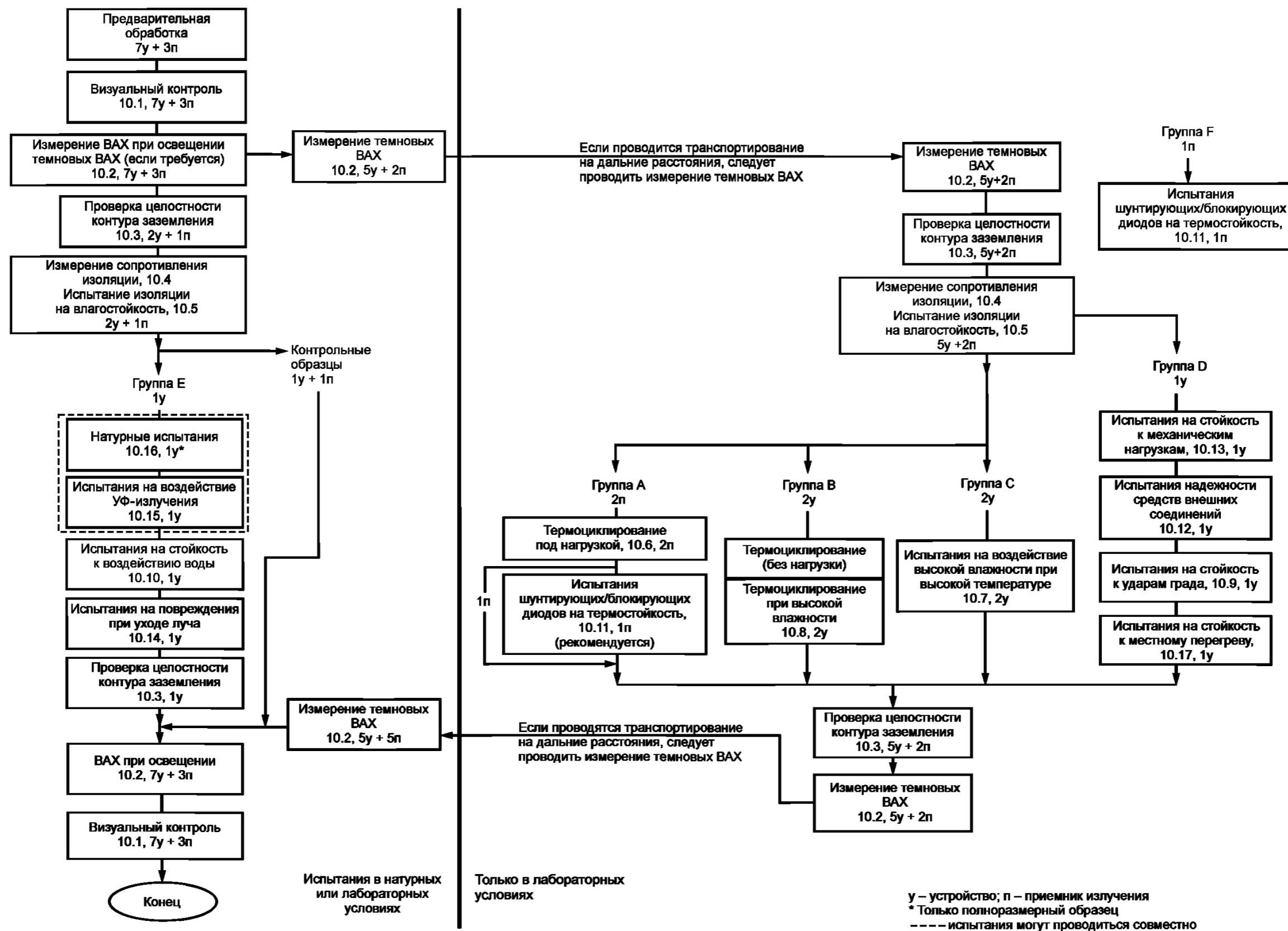
Рисунок 1 – Порядок проведения испытаний фотоэлектрических устройств с концентраторами, которые поставляются в готовом виде
