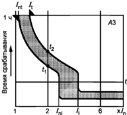
Рисунок А.3 — Характеристика тепловой и электромагнитной защиты
