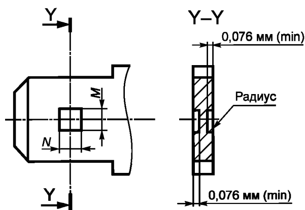
Рисунок Е.7 — Размеры круглых углублений фиксации (см. рисунок Е.6)
