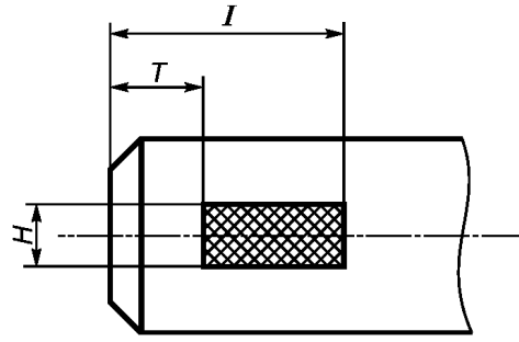
Рисунок E.10 — Размеры штыревого наконечника
