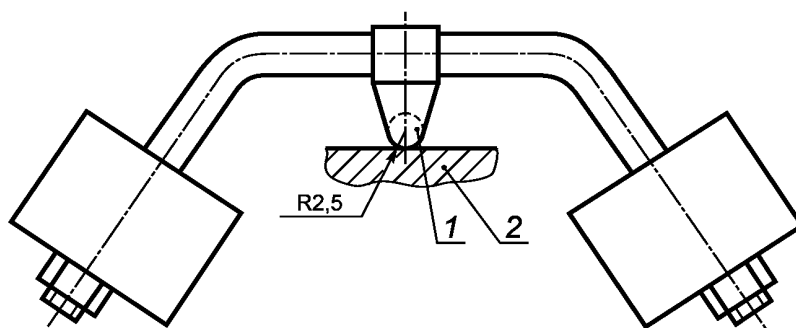
Рисунок 8 — Установка для испытаний давлением шарика
