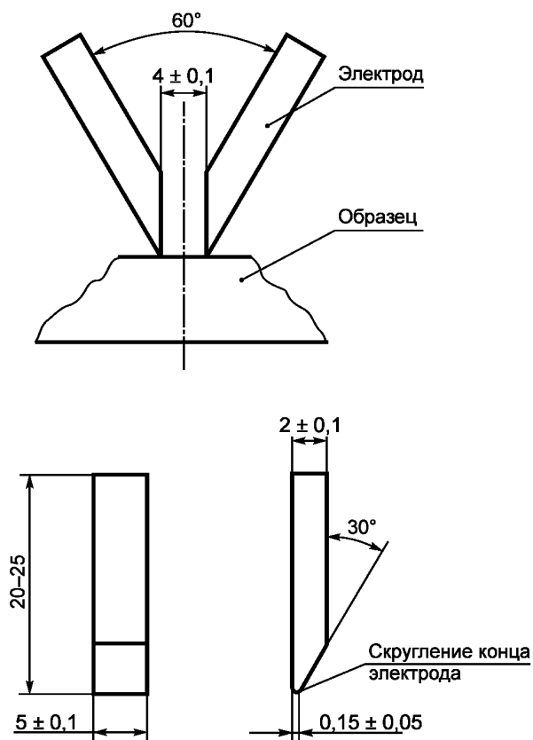
Рисунок 9 — Расположение и размеры электродов для испытания на трекингостойкость
