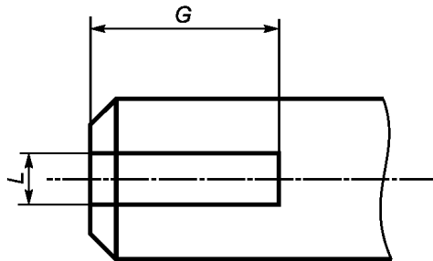
Рисунок E.11 — Размеры штыревого наконечника
