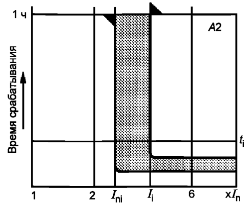
Рисунок А.2 — Характеристика только электромагнитной защиты
