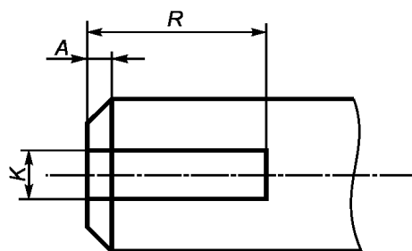
Рисунок E.12 — Размеры штыревого наконечника
