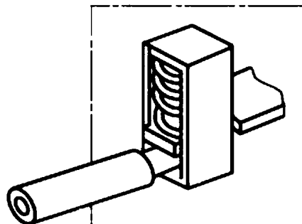
Безвинтовой вывод с непрямым зажимом
