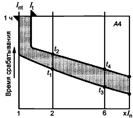
Рисунок А.4 — Характеристика гидравлическо-электромагнитной защиты
