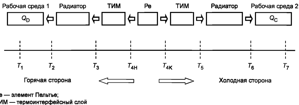
Рисунок 2 — Тепловые сопротивления
