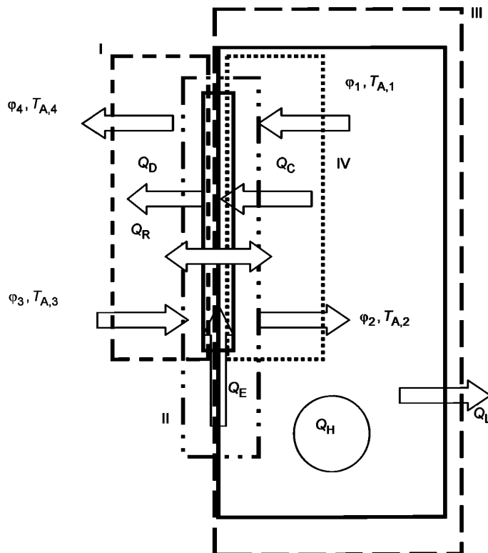
Рисунок 3 — Границы разделов термодинамической установки термоэлектрической системы охлаждения, присоединенной к закрытому шкафу
