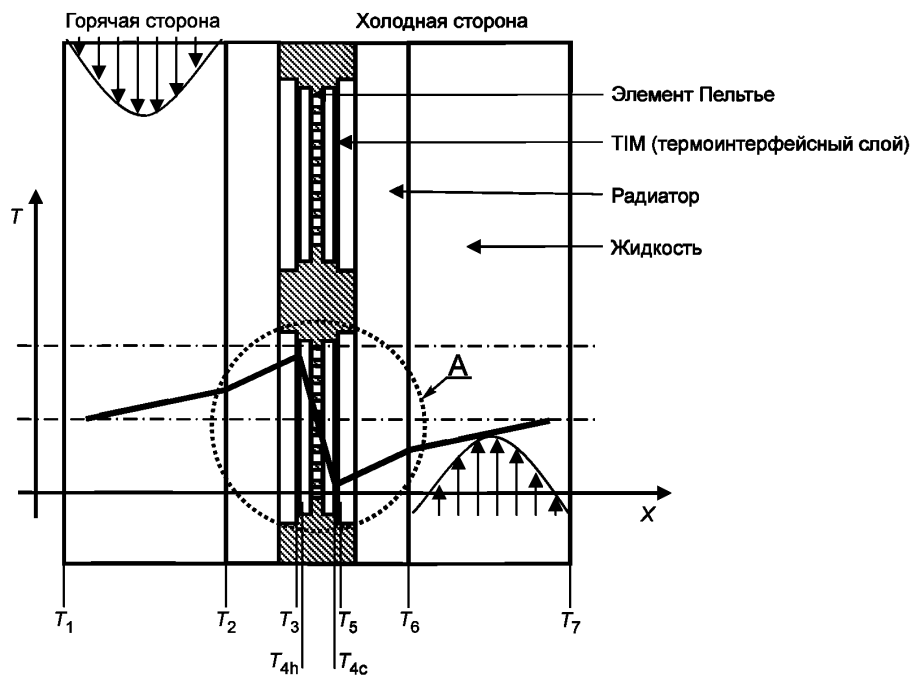
Рисунок 1, лист 1 — Принцип действия термоэлектрической системы охлаждения
