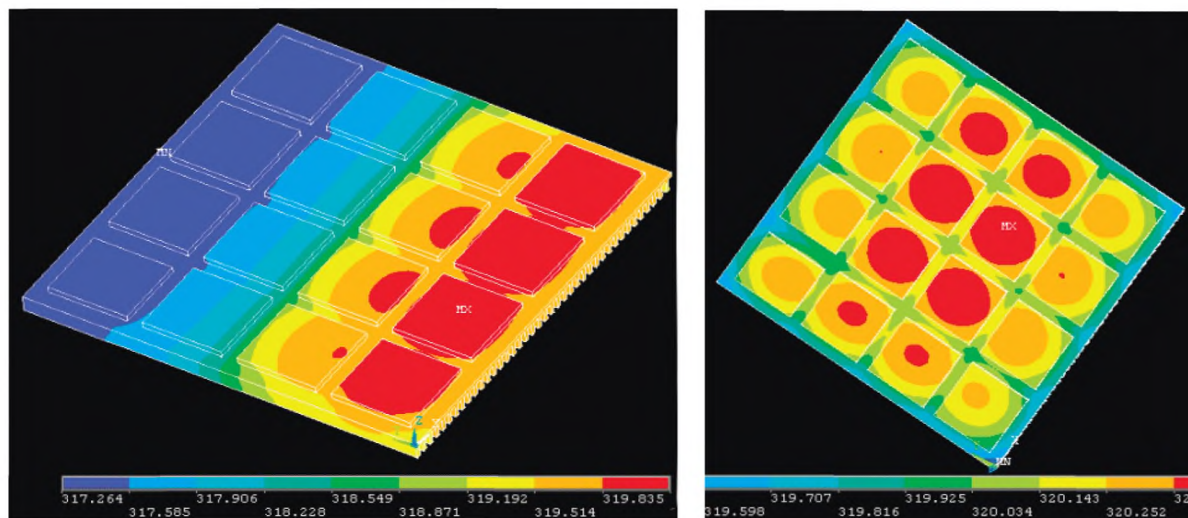
Рисунок А.9 — Распределение температуры общего тепловода при заданных граничных условиях
