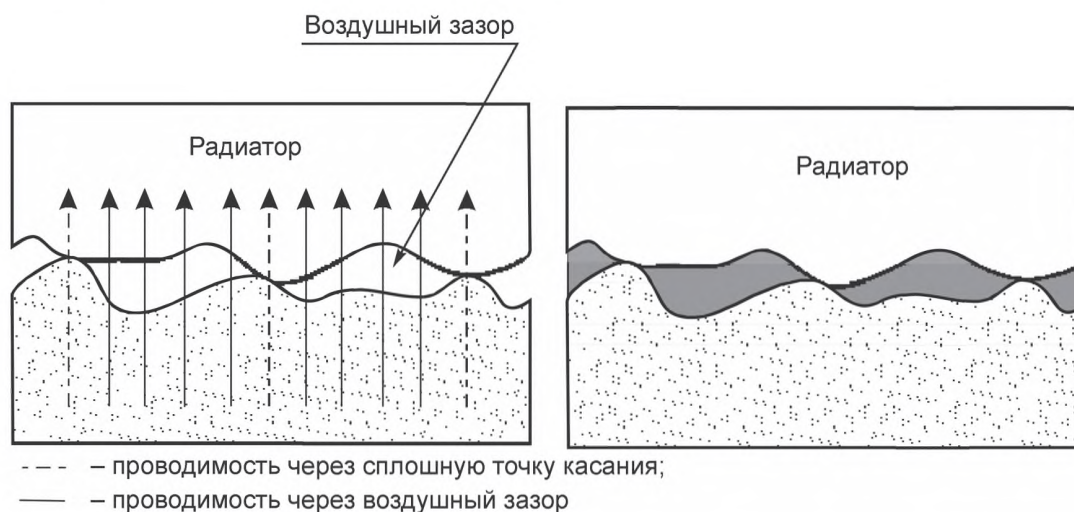
Рисунок А.10 — Графическое изображение значения слоя термоинтерфейса (ТИМ)
