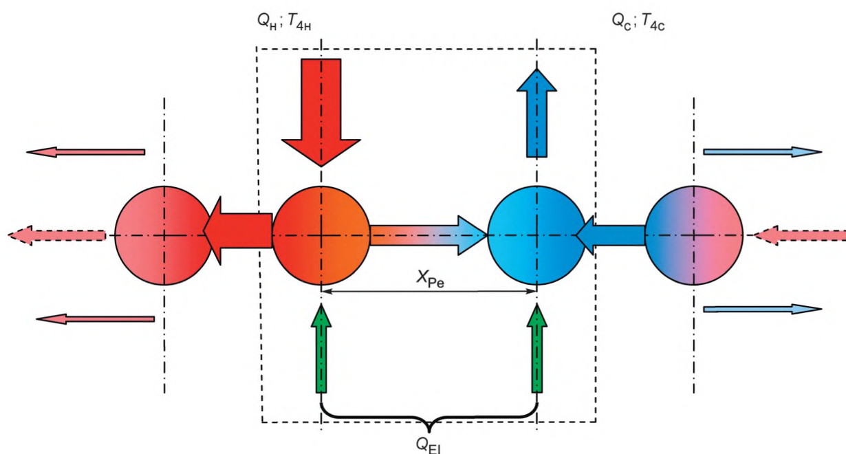
Рисунок А.5 — Границы разделов термодинамической установки элемента Пельтье
