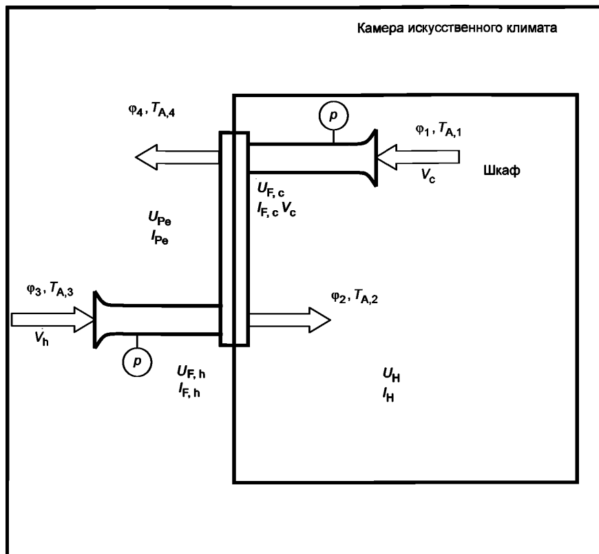
Рисунок 4 – Схема измерительной установки
