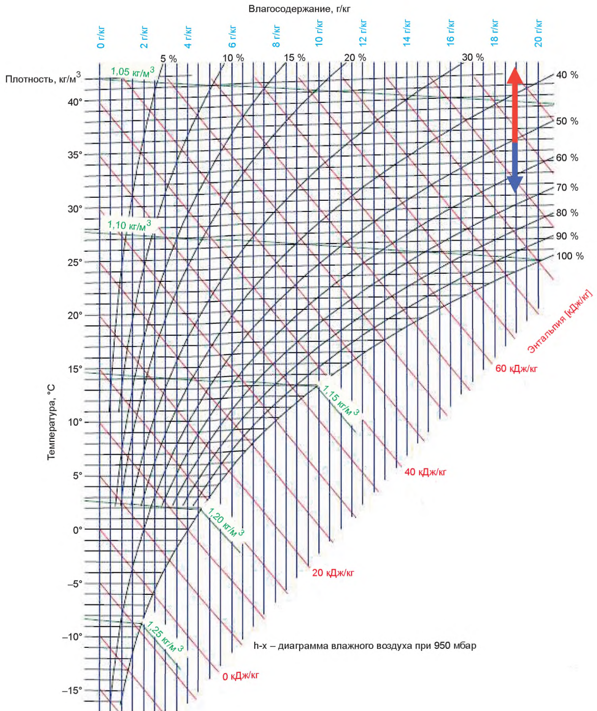
Рисунок А.1 — h-x — диаграмма Моллье для влажного воздуха
