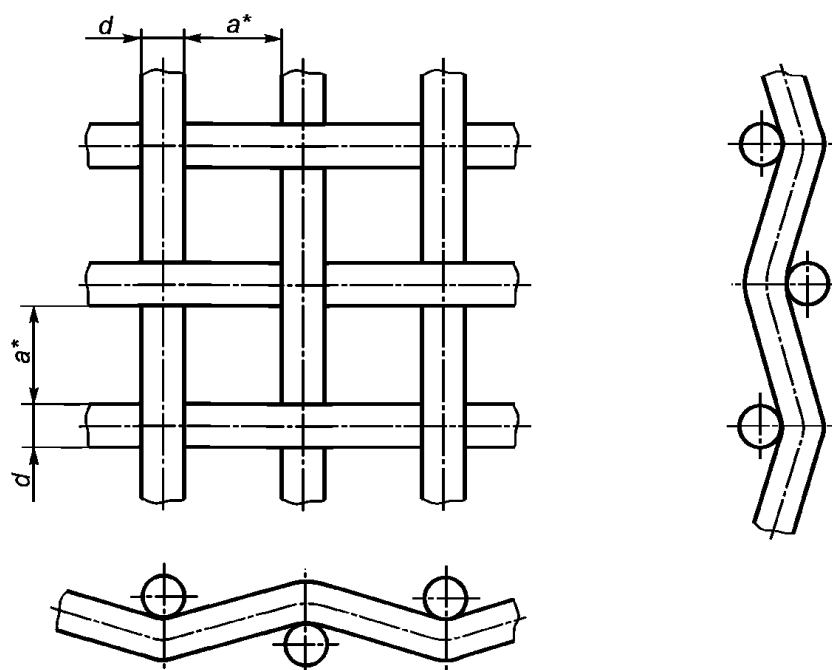
Рисунок 1 — Сетка типа ТК
