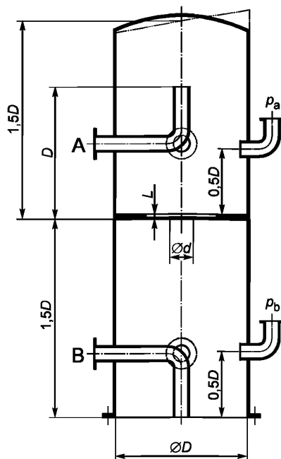
Рисунок 2 — Измерительная камера
