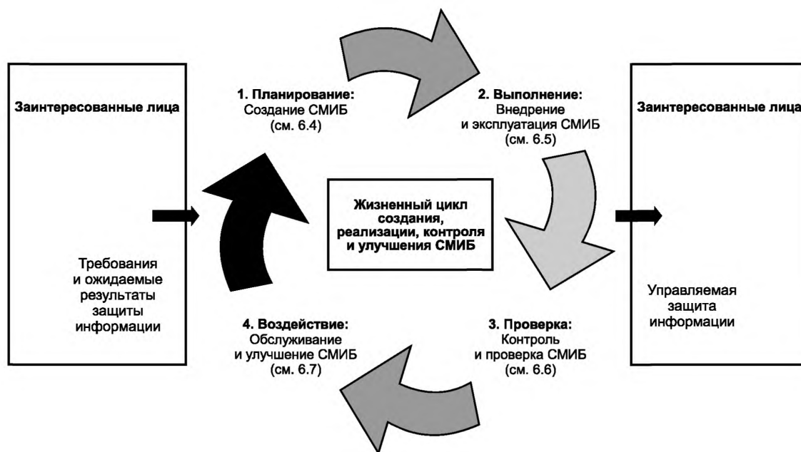
Рисунок 2 — Обзор системы менеджмента информационной безопасности
