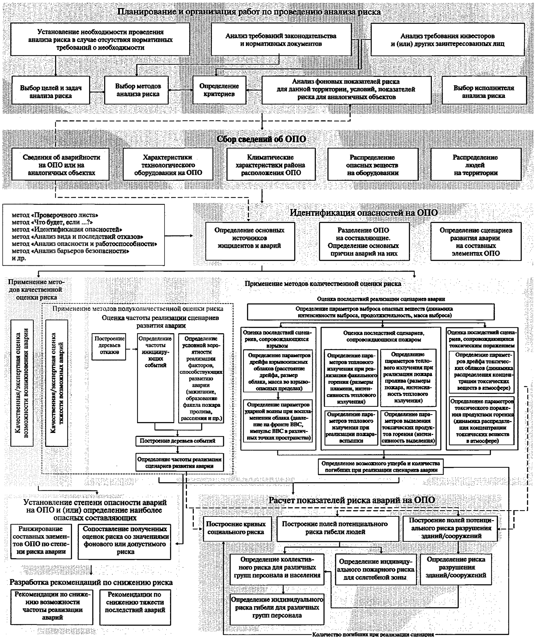
Рис. 3-1. Рекомендуемая схема анализа опасностей и оценки риска аварий, связанных с выбросом опасных веществ на ОПО
