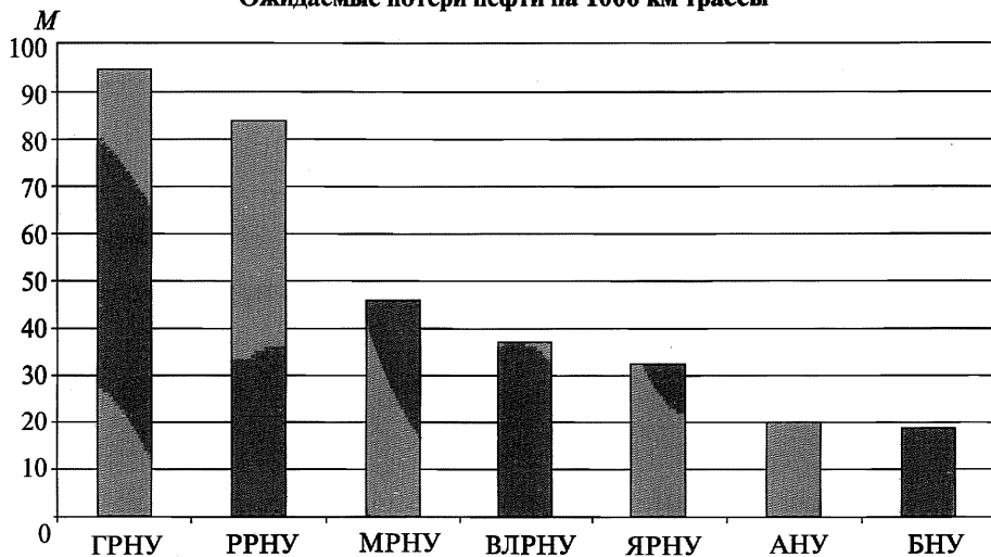
Рис.8-4.2 Ранжирование ОПО по удельным материальным потерям нефти
