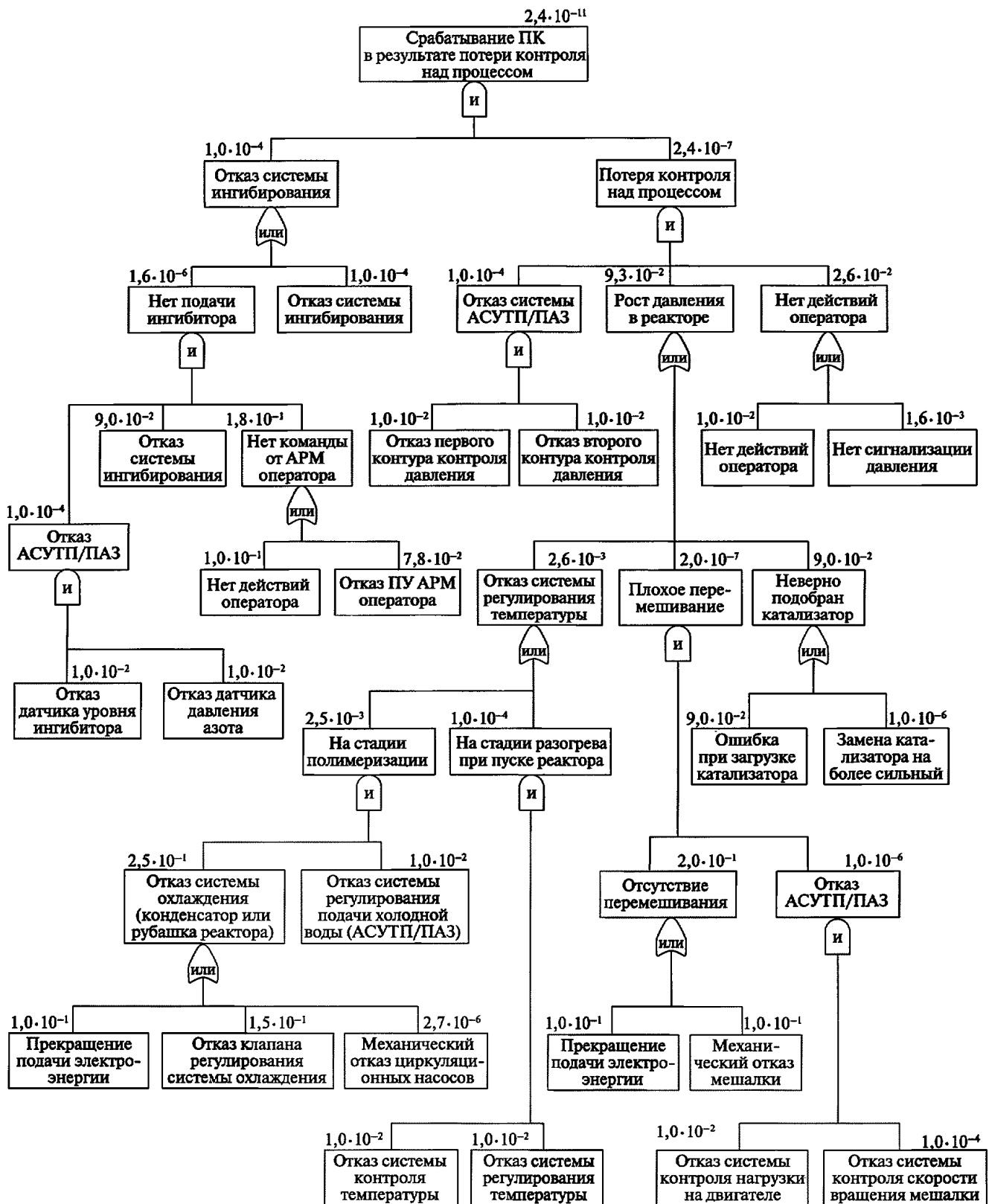
Рис. 8-1. Пример дерева отказов для химических реакторов
