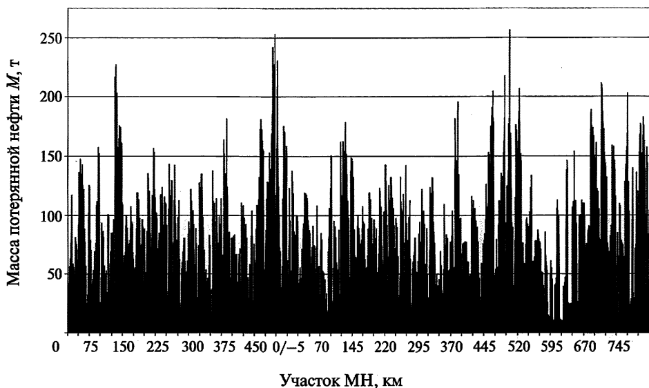
Рис. 8-4.1. Пример распределения показателя риска по трассе магистрального нефтепровода (км) и ранжирования ОПО
