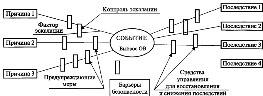
Рис. 8-3. Пример отображения применения метода АББ
