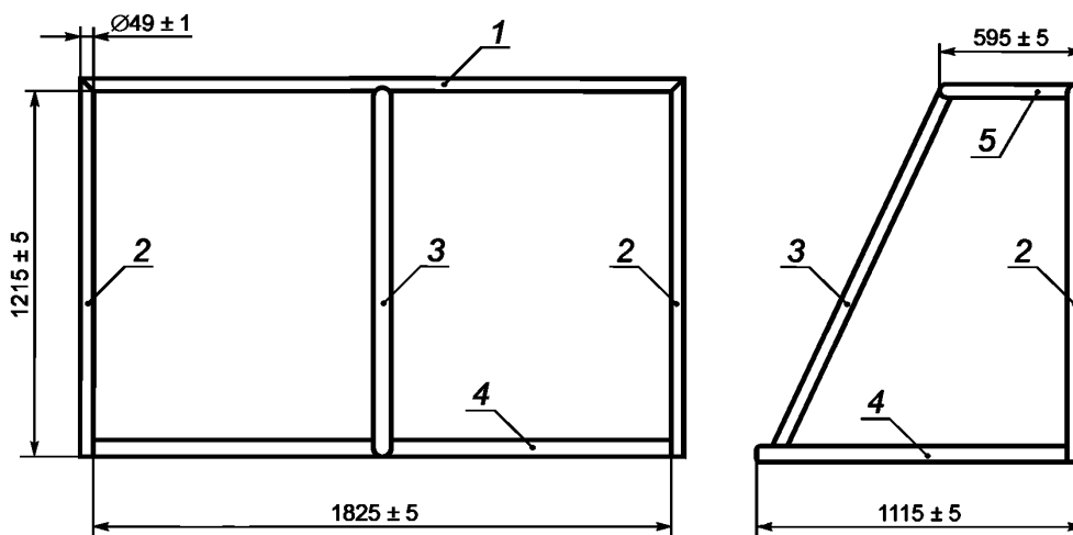
1 — перекладина; 2 — стойка; 3 — задняя стойка; 4 — нижняя рамка; 5 — верхняя рамка
