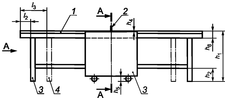
а) Вид сбоку
