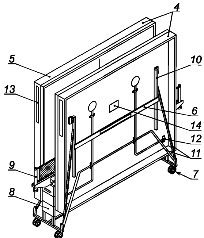
б) В положении для хранения
