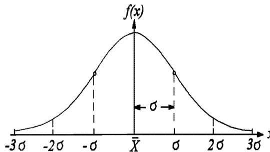
Рисунок П.8 – Кривая нормального распределения.
