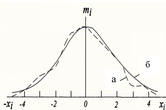
Рисунок П.2 – Полигон (1) и кривая распределения (2).
