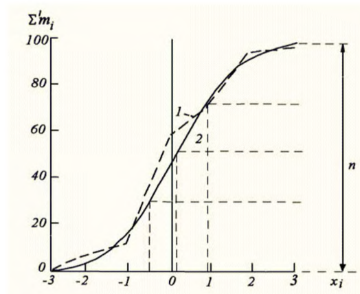
Рисунок П.3 – Оги́ва (1) и интегральная кривая распределения (2).
