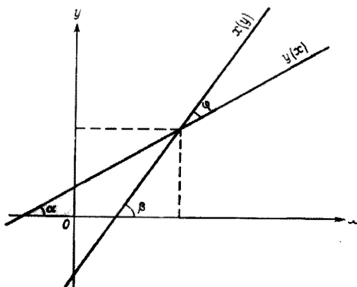
Рисунок П.10 – Прямые регрессии x(y) и y(x) .
