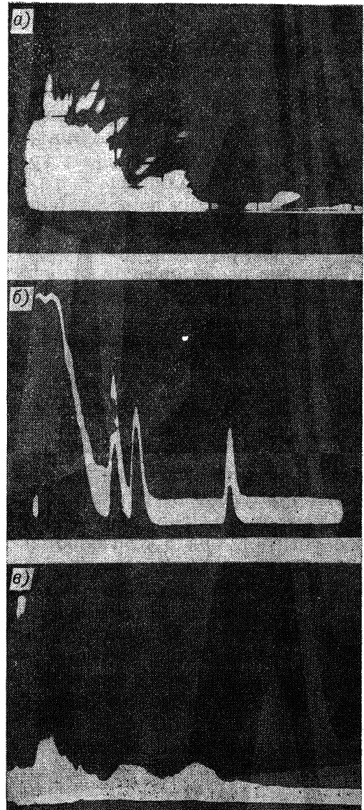
Черт. 2.21. Дискретно-когерентное радиоэхо.
