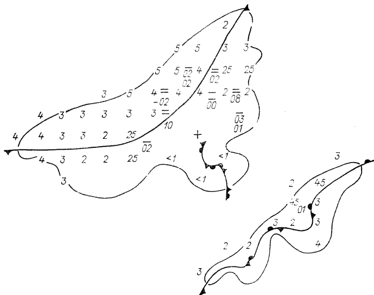
Черт. 5.8. Радиозеха облачности и осадков за 09 час 20 апреля 1981 г. Район Балхаша.
