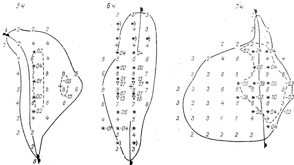
Черт. 5.3. Радиоэхо облачности и осадков теплого фронта, перемещающегося к востоку, за 28 января 1987 г.
