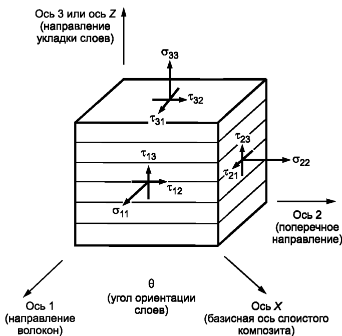
Рисунок 1 — Система координат материала
