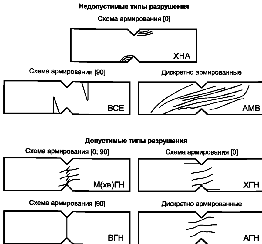
Рисунок 8 — Примеры обозначения типовых разрушений
