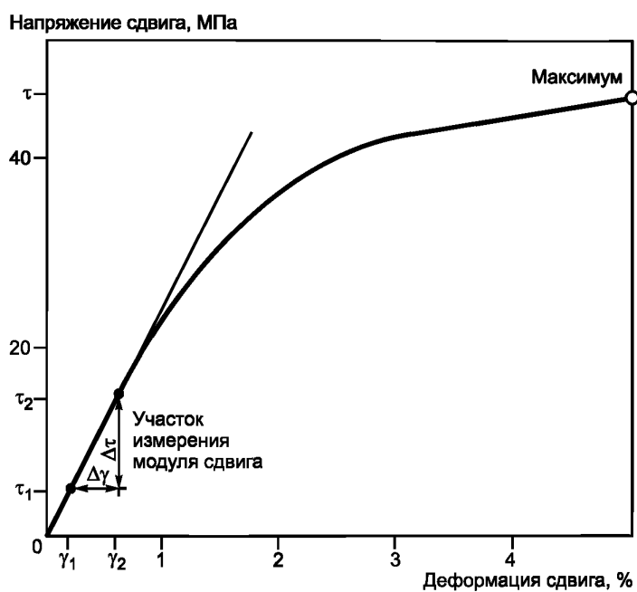
Рисунок 7 — Типовая диаграмма испытания на сдвиг образца с V-образным надрезом
