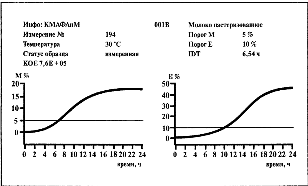
Рис. 4. Типичная кривая импедансного сигнала при определении КМАФАнМ с использованием питательной среды ViMedia 001В
