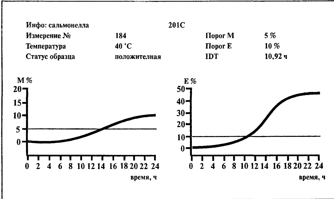
Рис. 6. Типичная кривая импедансного сигнала при определении сальмонелл с использованием питательной среды ViMedia 201С
