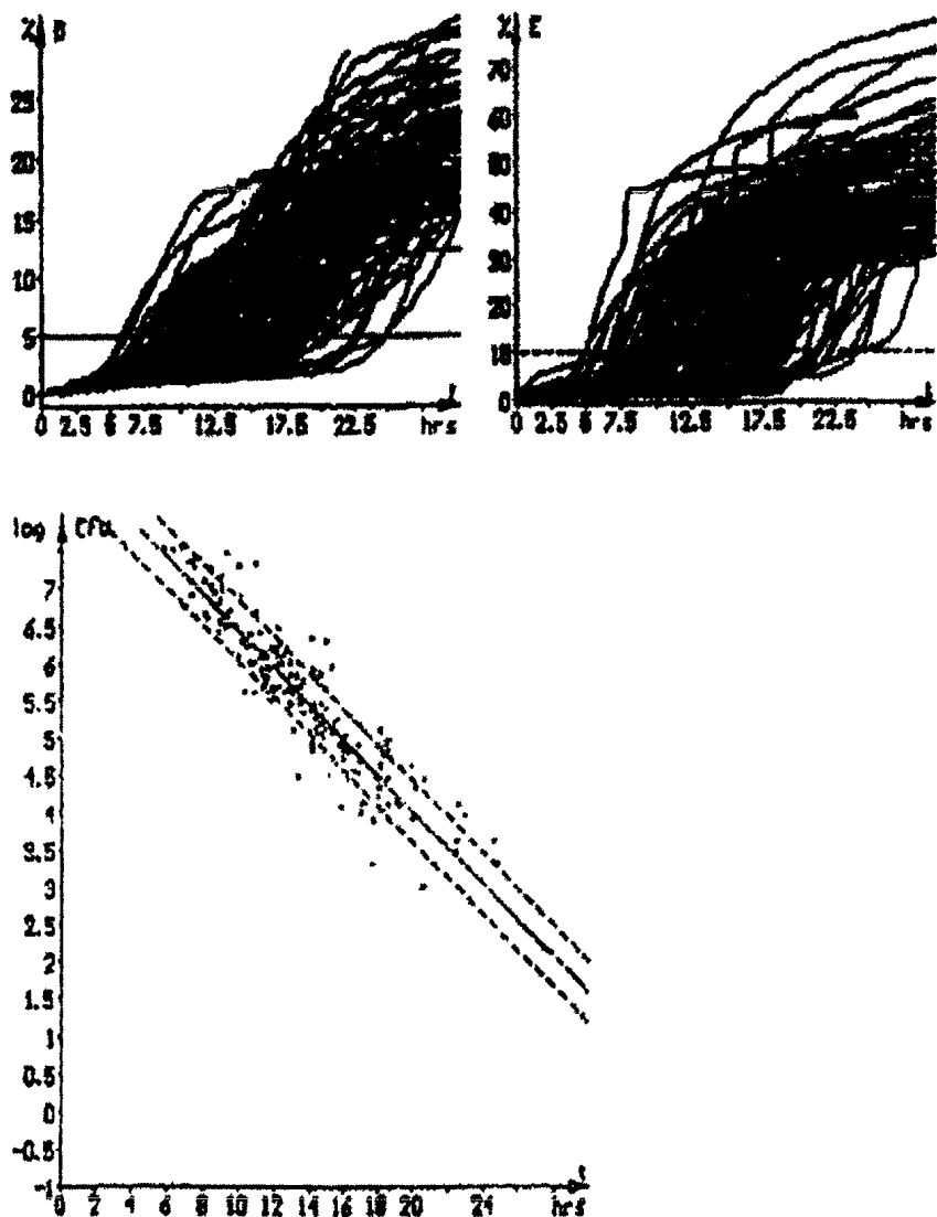
Рис. 3. Корреляция между логарифмом численности микроорганизмов \log КОЕ и временем определения импеданса t для образцов молока с использованием среды BiMedia 001B
