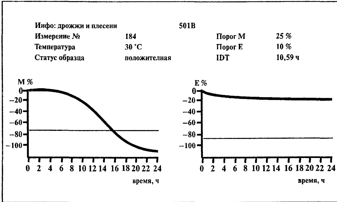
Рис. 10. Типичная кривая импедансного сигнала при определении дрожжей и плесеней с использованием питательной среды ViMedia 501B
