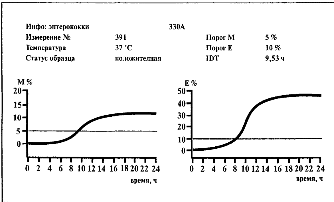
Рис. 7. Типичная кривая импедансного сигнала при определении энтерококков с использованием питательной среды BiMedia 330A
