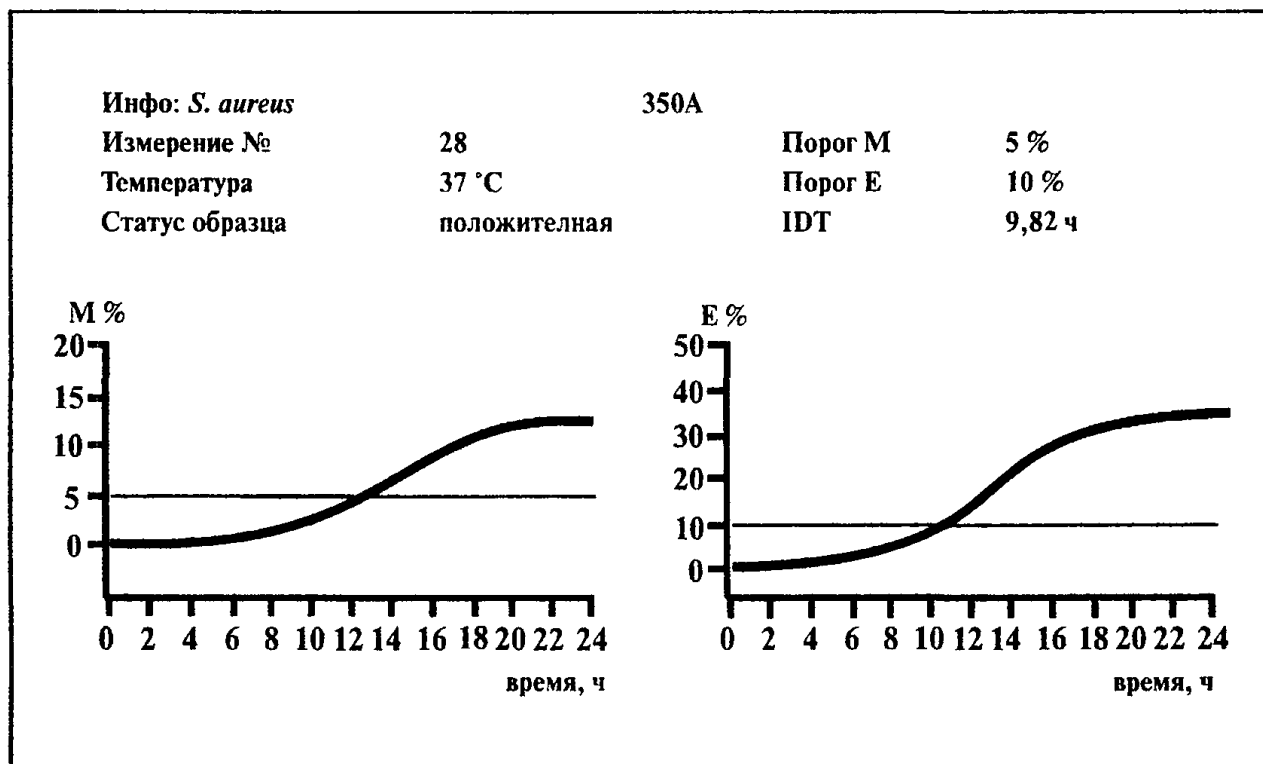
Рис. 8. Типичная кривая импедансного сигнала при определении S. aureus с использованием питательной среды BiMedia 350A
