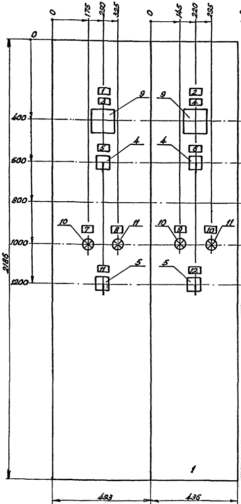
Левая и правая двери шкафа панели 1 Вид спереди М 1:10 Левая и правая двери шкафа панели 2 Вид спереди М 1:10
