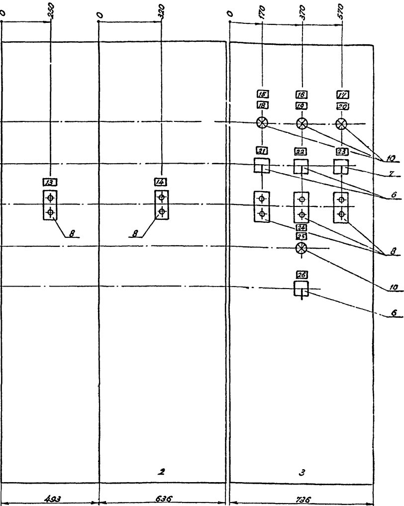
Левая и правая двери шкафа панели 1 Вид спереди М 1:10 Левая и правая двери шкафа панели 2 Вид спереди М 1:10
