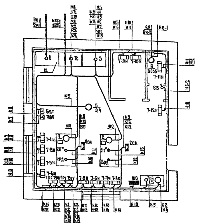
План насосной станции М 1:50 (с электроотоплением)
