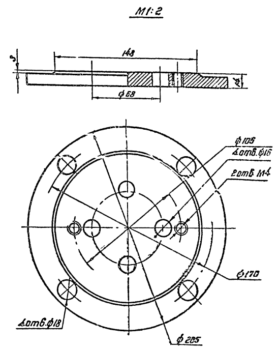
Крышка (поз. 1)
