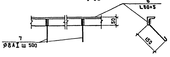
3A-2 1:10
