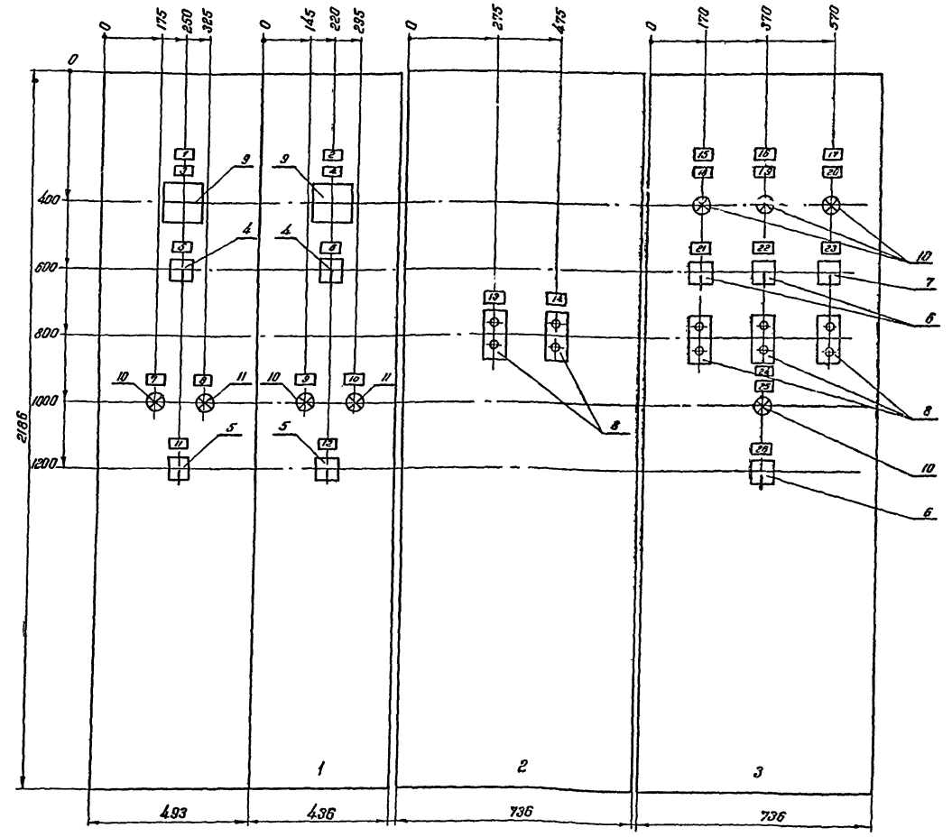
Левая и правая двери шкафа панели 1 Вид спереди м1:10 Дверь шкафа панели 2 Вид спереди м1:10 Дверь шкафа панели 3 Вид спереди м1:10
