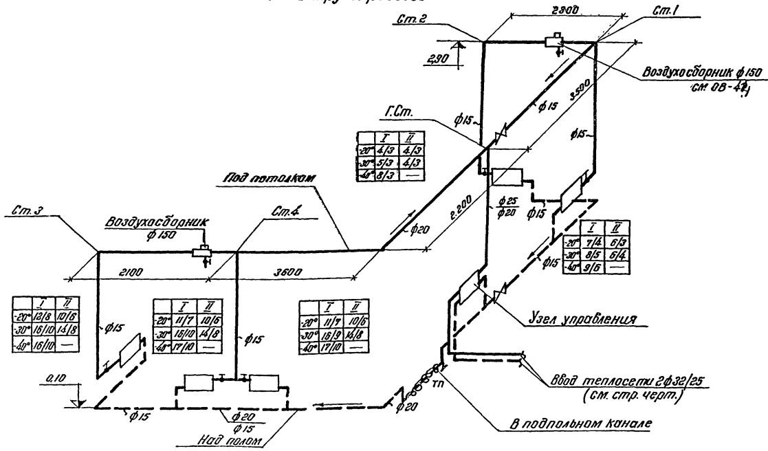
Схема трубопроводов
