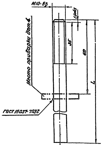
Электрод (поз. 6)
