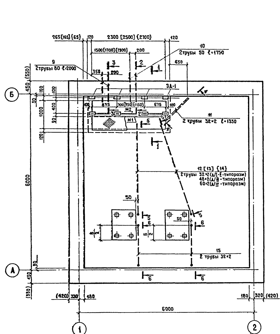
3A-1 1:10
