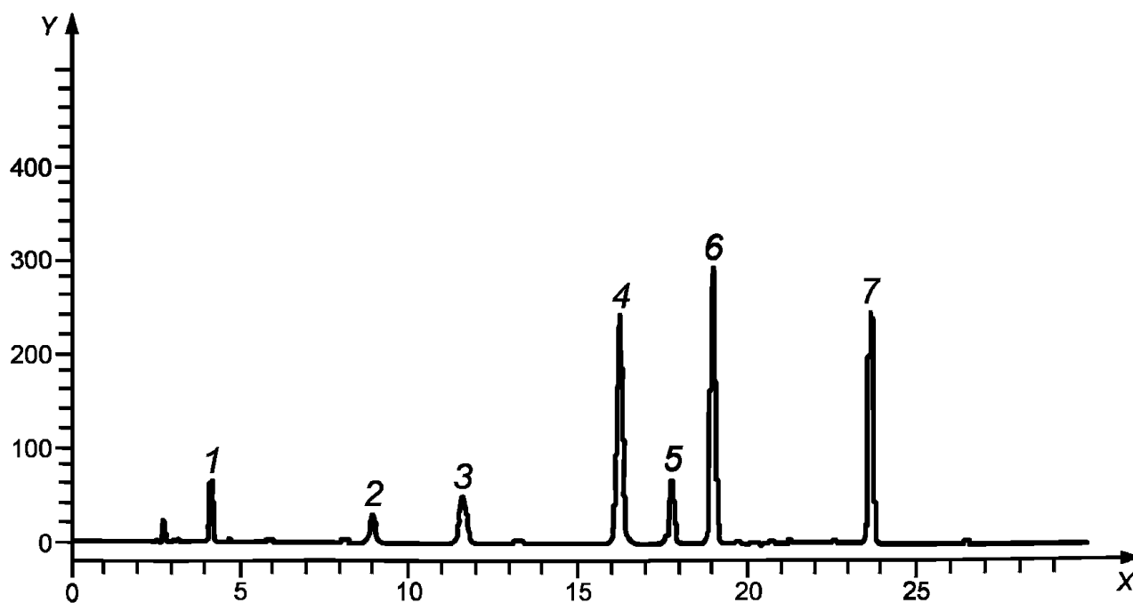
X — время удерживания, мин; Y — отклик, mAU; 1 — галловая кислота; 2 — EGC; 3 — катехин; 4 — кофеин; 5 — эпикатехин; 6 — EGCG; 7 — ECG
