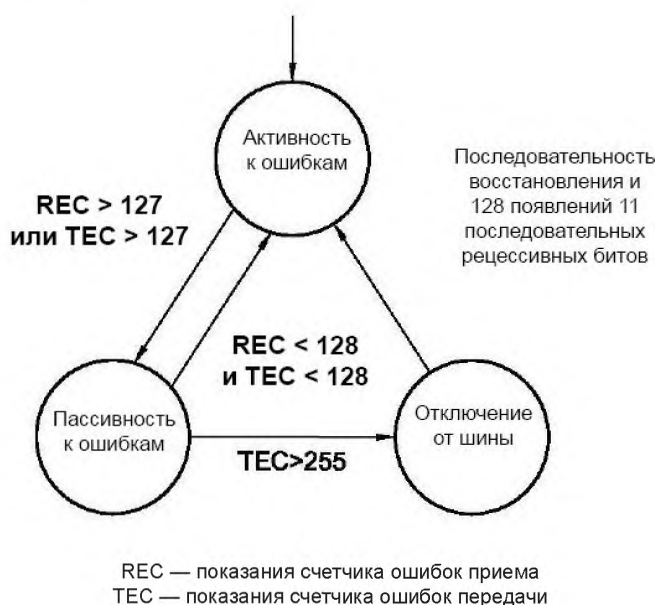
Рисунок 16 — Схема смены состояния узла
