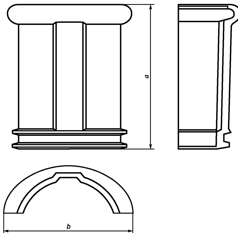
Рисунок А.4 — Коньковая черепица
