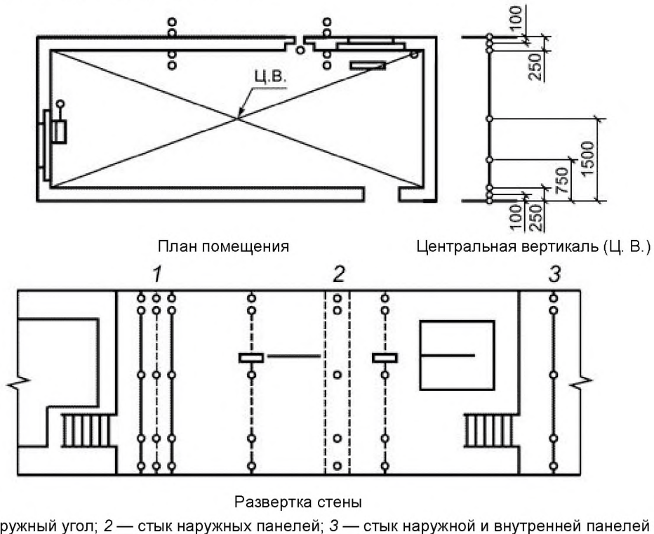
Рисунок А.1 — Схема размещения термодатчиков на испытываемой ограждающей конструкции и подключения их к измерительной аппаратуре
