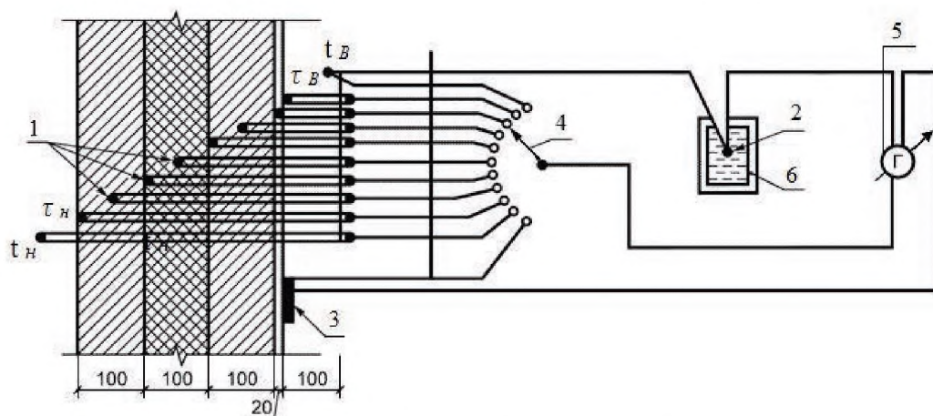
Рисунок А.1 — Схема размещения термодатчиков на испытываемой ограждающей конструкции и подключения их к измерительной аппаратуре
