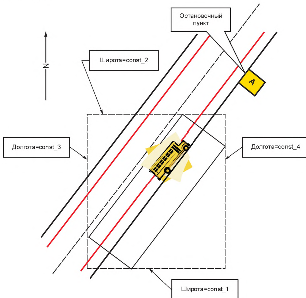
Рисунок 2 — Схема организации пространственной модели участка
