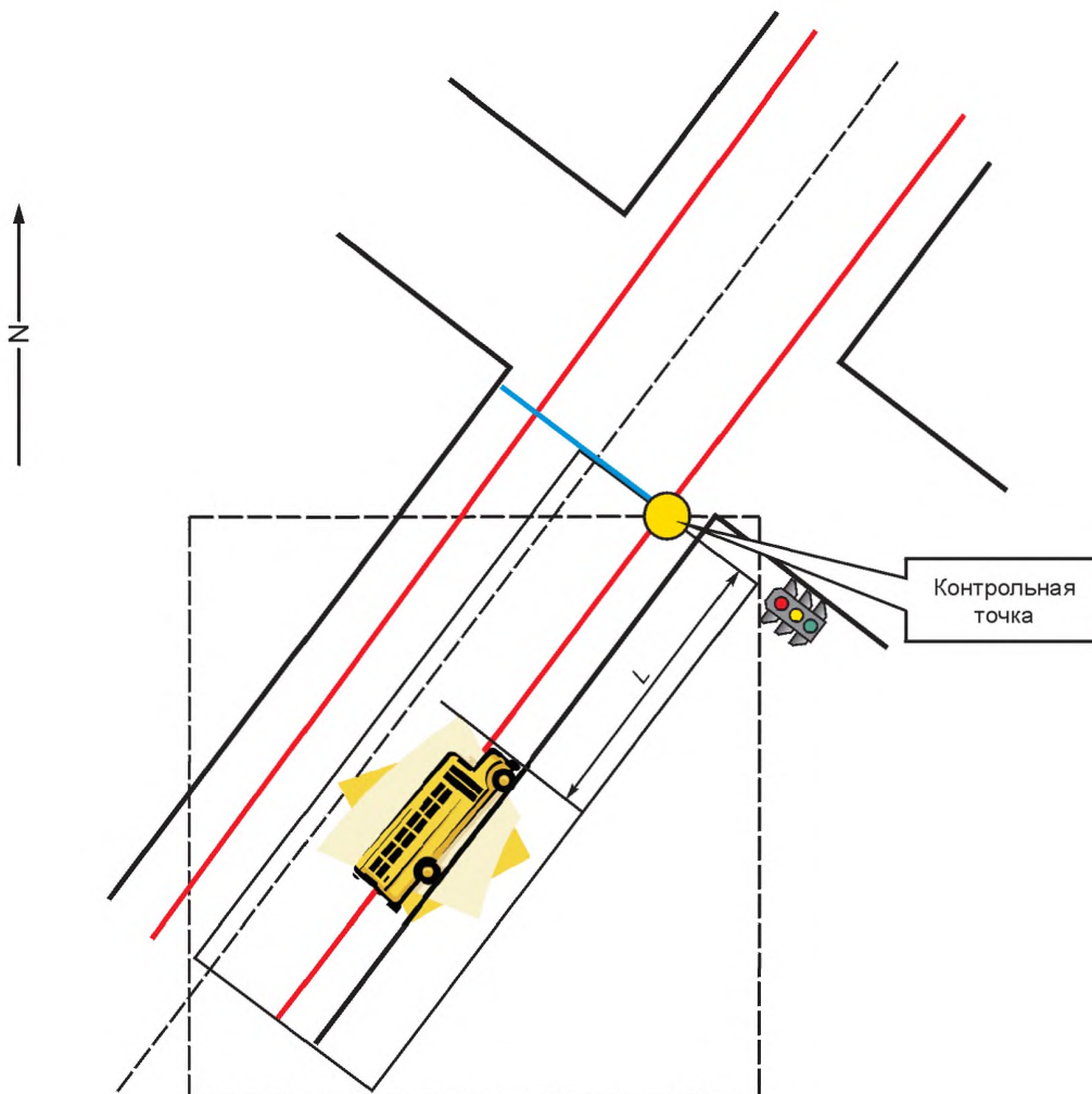
Рисунок 4 — Схема организации пространственной модели регулируемого перекрестка
