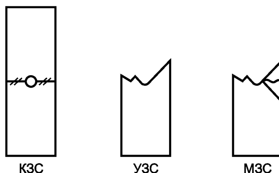
Рисунок 2 — Примеры допустимых типов разрушения
