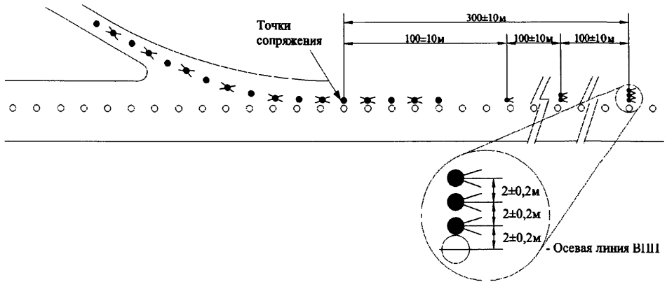
Рисунок 13. Огни указателя РД быстрого схода с ВПП.
