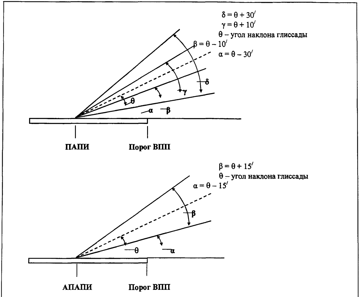
Рисунок 15. Углы возвышения огней в системах PAR I и APAR I (для углов наклона глиссады 2^{\circ} - 4^{\circ} )
