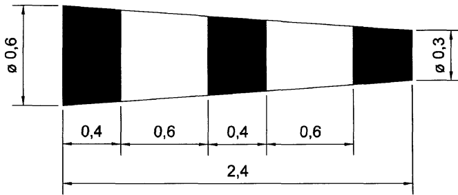
Рисунок. Конус-ветроуказатель
